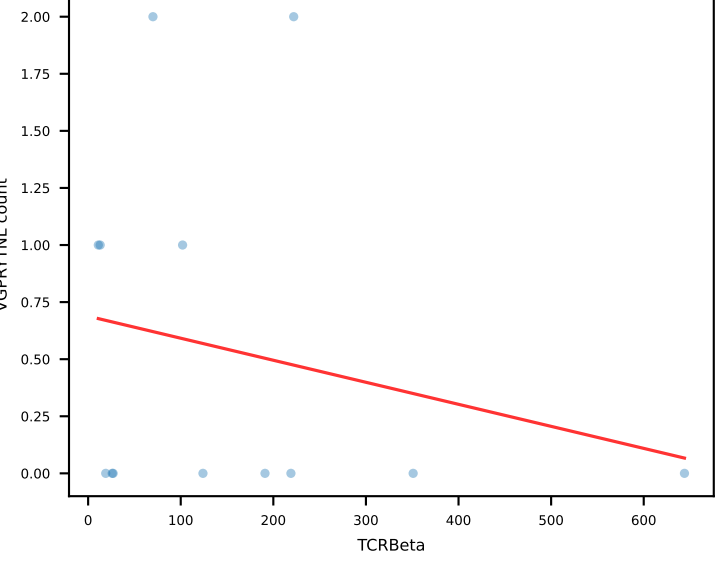
VGPRYTNL r=-0.22 p=0.46
