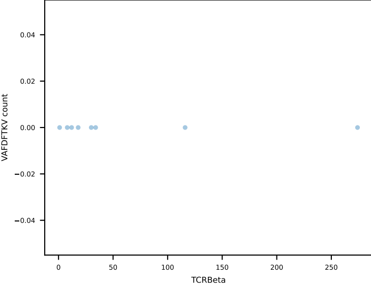
VAFDFTKV
