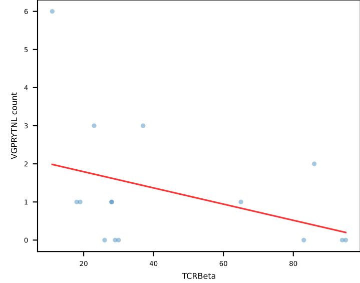
VGPRYTNL r=-0.39 p=0.15
