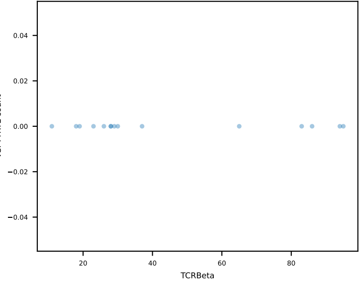
VSFTYRYL
