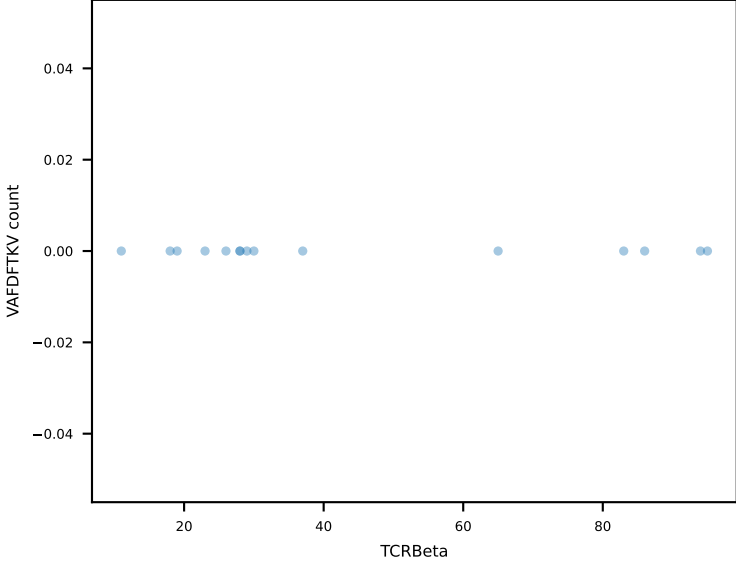
VAFDFTKV
