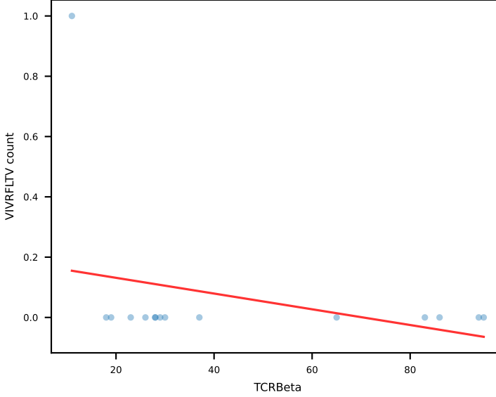
VIVRFLTV r=-0.31 p=0.27
