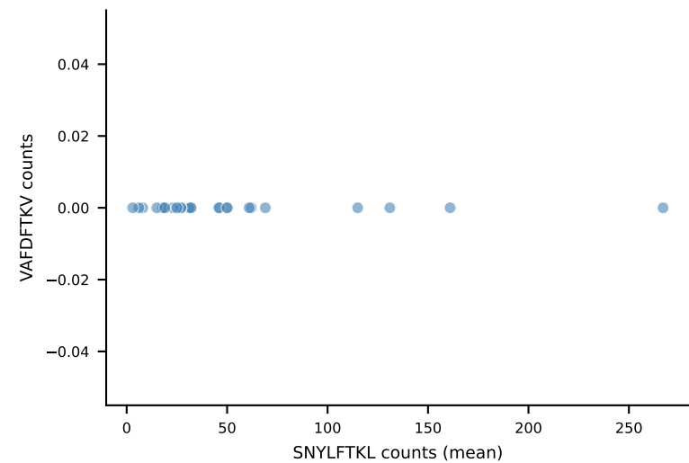
SYFPEITHI r=-0.031 , p=8.81e-01
