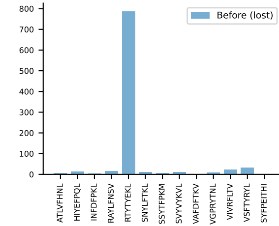
AV6-1-CVLGDGGSGNKLIf-AJ32_BV3-CASSLGvQDTQYf-BJ2-5- AV6-1-CVLGDGGSGNKLIf-AJ32_BV3-CASSLGvQDTQYf-BJ2-5 RAW n:6→0 LOST
