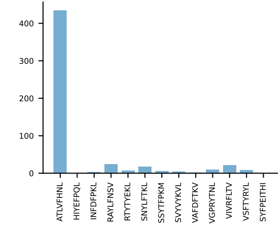
AV12-2-CALRASNTDKVfVf-AJ34*p03_BV1-CTCSADWDEQYf-BJ2-2AV12-2-CALRASNTDKVfVf-AJ34*p03_BV1-CTCSADWDEQYf-BJ2-2 RAW n:5→0 LOST
