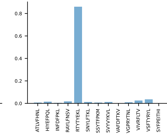
AV6-1-CVLGDGGSGNKLIf-AJ32_BV3-CASSLGvQDTQYf-BJ2-5 PROP n:6→0 LOST
