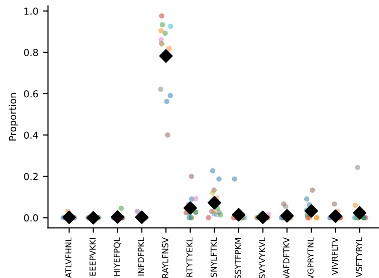
#102 AV8D-1-CATDGASSSFSKLTV-AJ50_BV1-CTCSADGVEQYF-BJ2-7 coh=0.940, n=12
