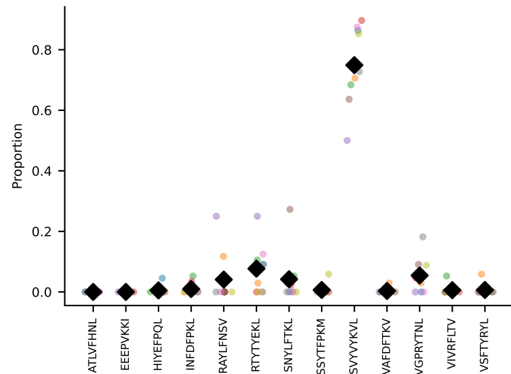
#106 AV8-1-CATDGASSSFSKLTV-AJ50_BV1-CTCSADGVEQYF-BJ2-7 coh=0.935, n=9
