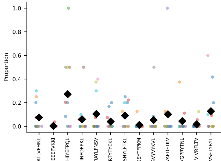
#65 AV13-2-CAIDPNYNVLYF-AJ21_BV13-3-CASSDWGNYAEQFF-BJ2-1 coh=0.273, n=5
