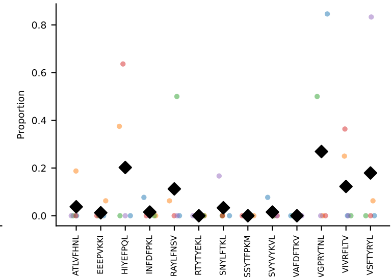
#128 AV10N-CAASMAGGNYPKF-AJ6_BV1-CTCSADSGGNYPKF-BJ2-2 coh=0.171, n=9
