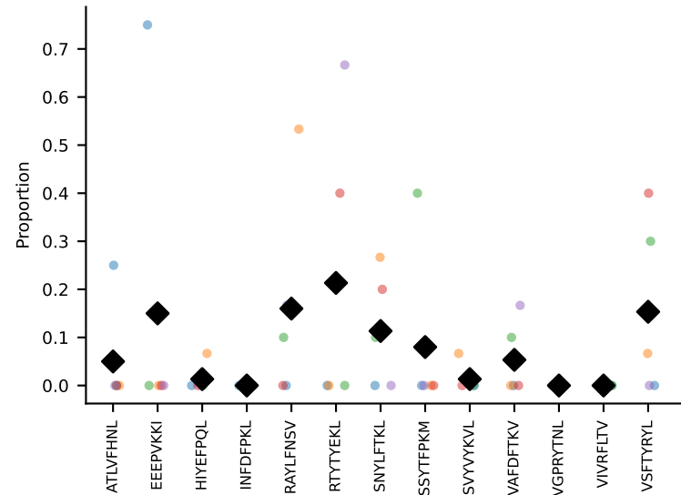
#126 AV10-CAASIASSSF SKLVF-AJ50_BV1-CTCSATNNQAPLF-BJ1-5 coh=0.173, n=8
