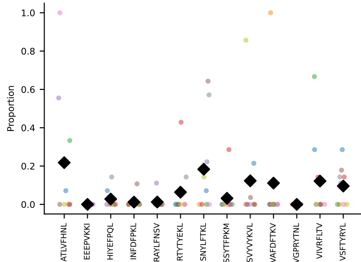
#144 AV7D-5-CAVKGQGTGSKLSF-AJ58_BV1-CTCSATGGGNQAPLF-BJ1-5 coh=0.190, n=13
