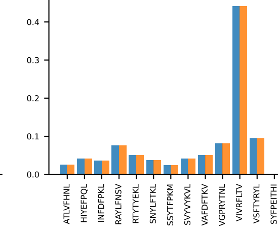
AV5-1-CSASTGGFASALT-AJ35_BV2-CASSQDGAGANSDYTF-BJ1-1AV5-1-CSASTGGFASALT-AJ35_BV2-CASSQDGAGANSDYTF-BJ1-1 PROP n:6→6
