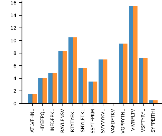
AV5-1-CSASTGGFASALT-AJ35_BV2-CASSQDGAGANSDYTF-BJ1-1AV5-1-CSASTGGFASALT-AJ35_BV2-CASSQDGAGANSDYTF-BJ1-1 MEAN n:6→6
