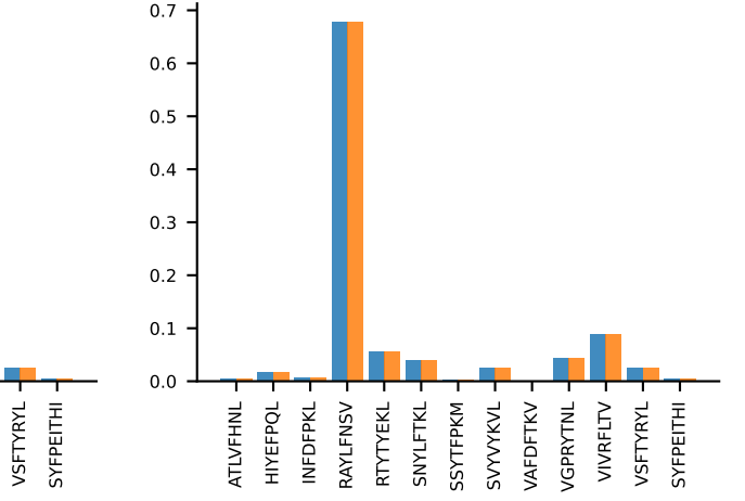
AV16D/DV11-CAMRDPYGGSGNKLIF-AJ32_BV1-CTCSAVREDTQYF-BJ2-2AV16D/DV11-CAMRDPYGGSGNKLIF-AJ32_BV1-CTCSAVREDTQYF-BJ2-2 PROP n:6→6
