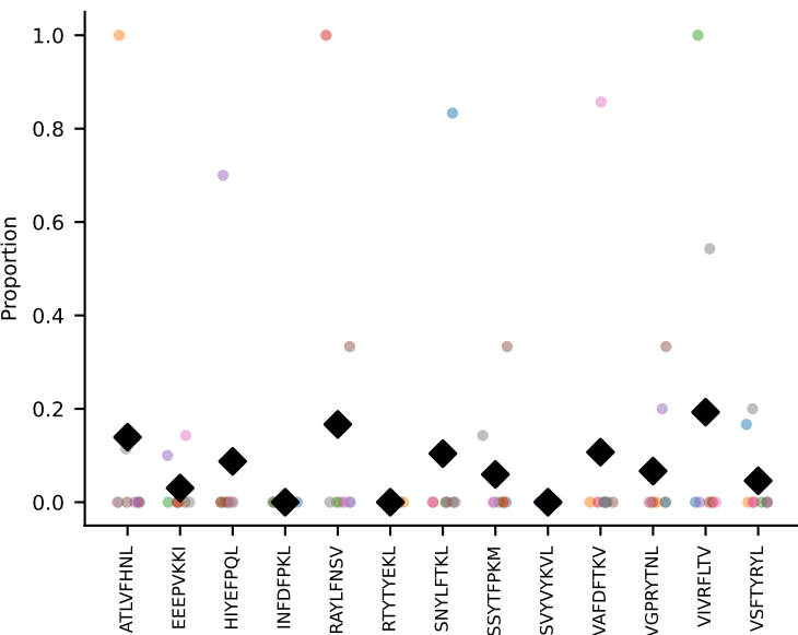
#65 AV6D-7-CALGGNYNQGLIF-AJ23_BV13-1-CASSDALYAEQFF-BJ2-1 coh=0.073, n=8
