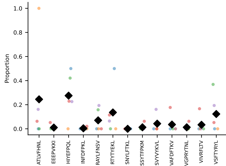
#19 AV12-2-CALNQGGSAKLIF-AJ57_BV1-CTCSADWGNIAEQFF-BJ2-1 coh=0.336, n=8
