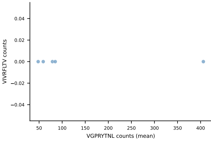
VIVRFLTV
