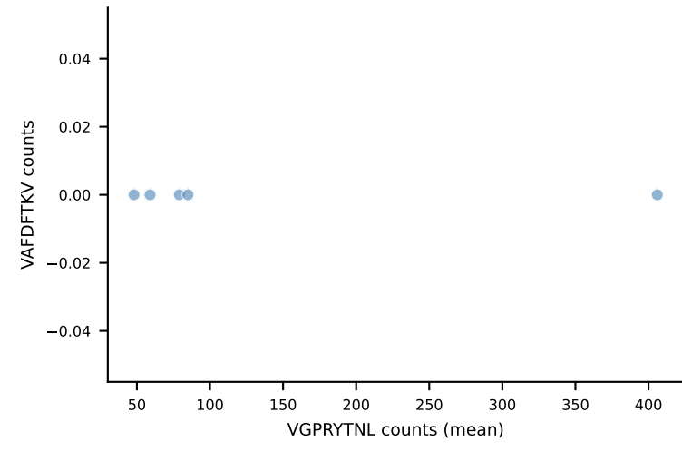
VAFDFTKV
