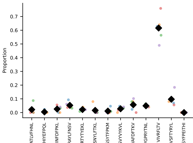
#33 AV14-3-CAASPNAVKVIF-AJ30_BV16-CASSFSGTGEYEQYF-BJ2-7 coh=0.969, n=5
