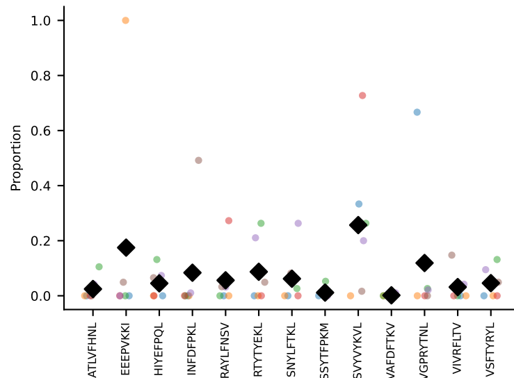
#56 AV19-CAEASSSFSKLVF-AJ50_BV16-CASSPRTGGYAEQFF-BJ2-1 coh=0.185, n=8
