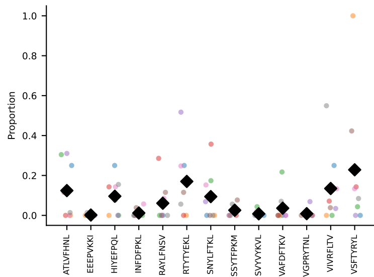
#31 AV4-3-CAATGGNNKLTf-AJ56_BV19-CASSIVSYAEQFF-BJ2-1 coh=0.355, n=5
