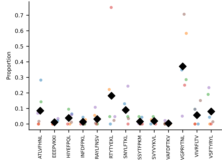
#17 AV3D-3-CAAPSNMGYKLTf-AJ9_BV5-CASSQGQGAEQFF-BJ2-1 coh=0.498, n=12
