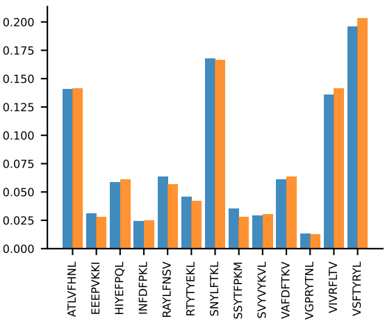
AV7N-4-CAVSEDRGSALGRLHF-AJ18_BV1-CTCSAGGDYAEQFF-BJ2-1 PROP n:19→7
