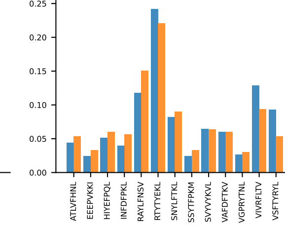
AV2-CIVTDMNYNQGLKIF-AJ23_BV19-CASSPTGPNSDYTF-BJ1-2 PROP n:16→10
