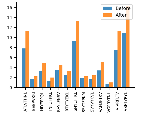
AV7N-4-CAVSEDRGSALGRLHF-AJ18_BV1-CTCSAGGDYAEQFF-BJ2-1 MEAN n:19→7
