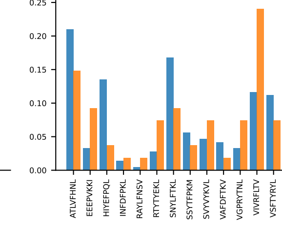
AV6-6-CALGDGTGGYKVVf-AJ12_BV14-CASSFWNYAEQFF-BJ2-1 PROP n:16→11
