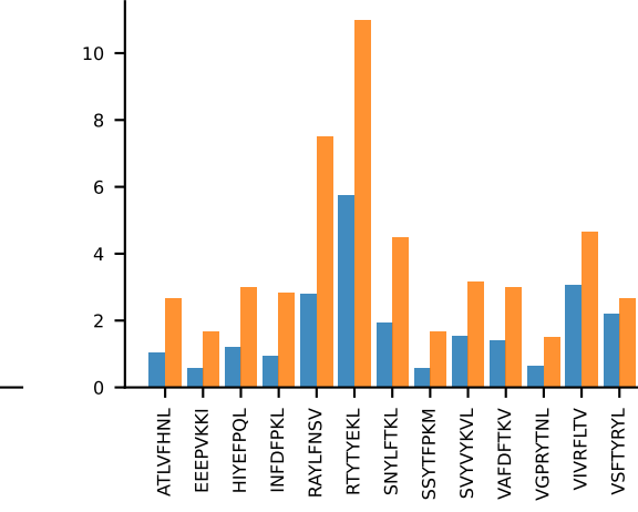
AV2-CIVTDMNYNQGLKIF-AJ23_BV19-CASSPTGPNSDYTF-BJ1-2 MEAN n:16→10
