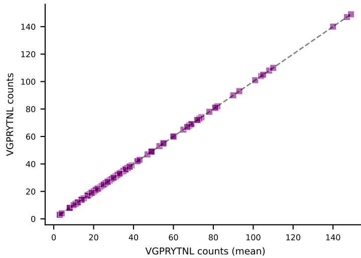
VGPRYTNL r=1.000 , p=0.00\text{e+}00
