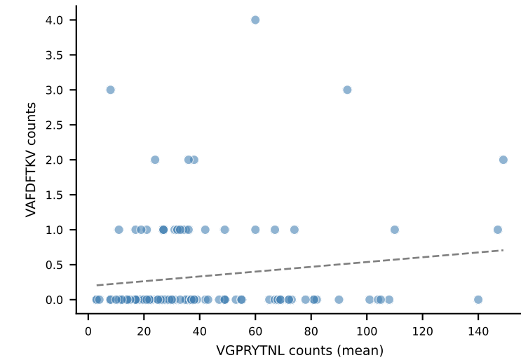
VAFDFTKV r=0.146 , p=1.18\text{e-}01
