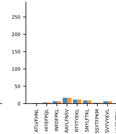
AV6-6-CALGTFSTNDKVVV-AJ34*p02_BV13-2-CASGTTYEQYF-BJ2-7 PROP n:17→17
