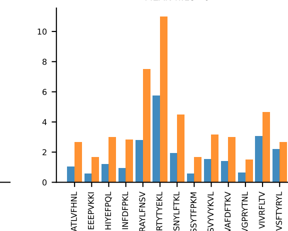
AV2-CIVTDMNYNQGLIF-AJ23_BV19-CASSPTGPNSDYTF-BJ1-2 MEAN n:16→10
