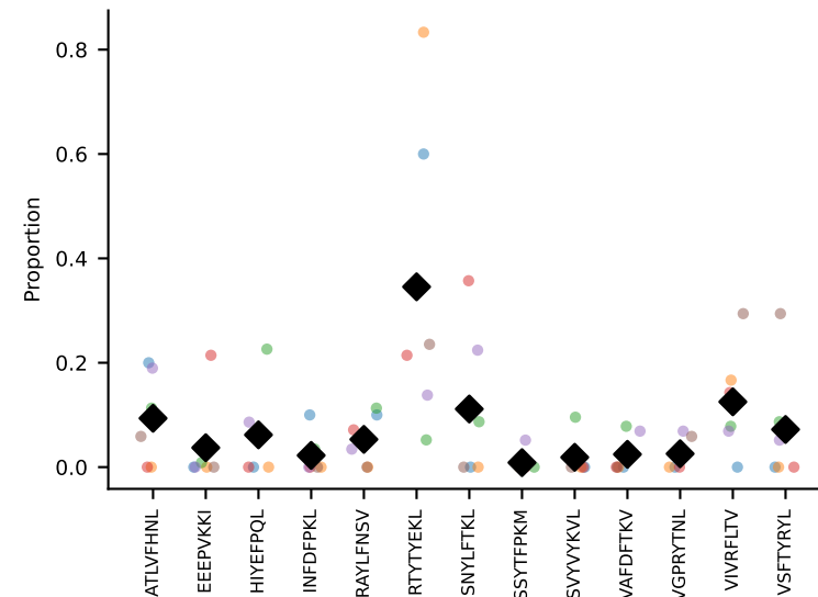
#17 AV13-1-CALEPSGSWQLIF-AJ22_BV1-CTCSAGTGGDTGQLYF-BJ2-2 coh=0.451, n=9
