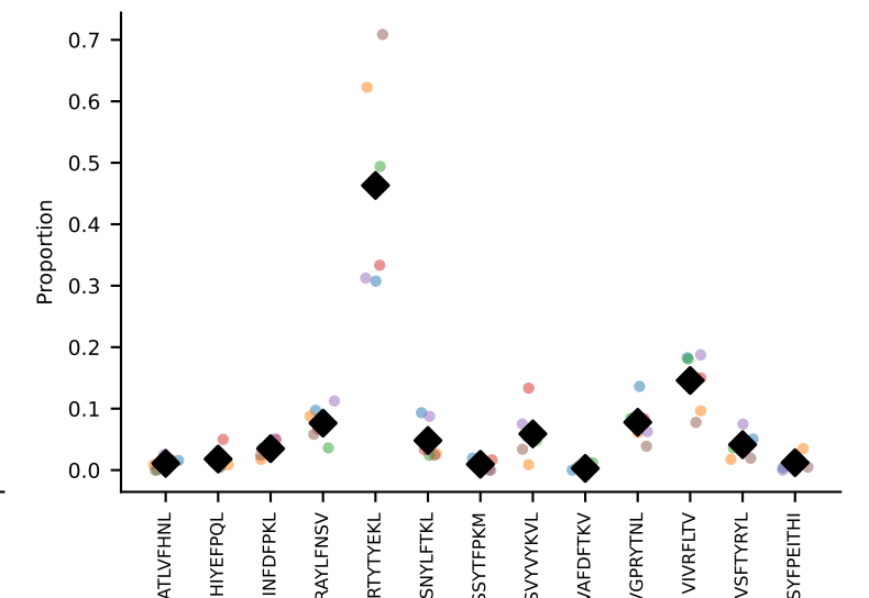
#68 AV16D/DV11-CAMREGMGYKLTFF-AJ9_BV13-2-CASGETNTEVFF-BJ1-3 coh=0.913, n=5
