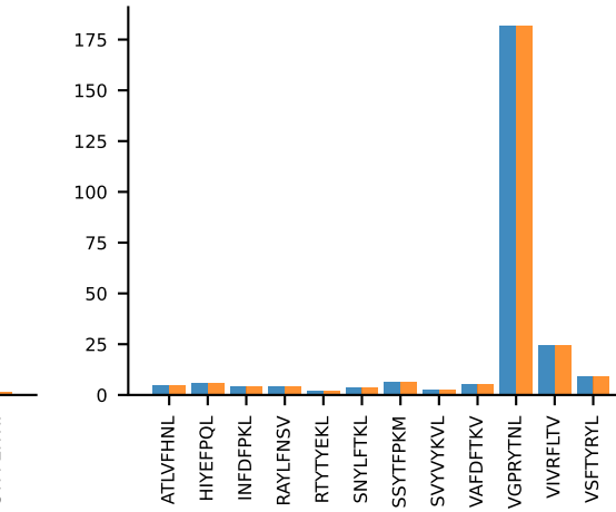
AV13D-1-CAMNQGGSAKLIF-AJ57_BV1-CTCSALNAYEQFF-BJ2-1 MEAN n:5→5
