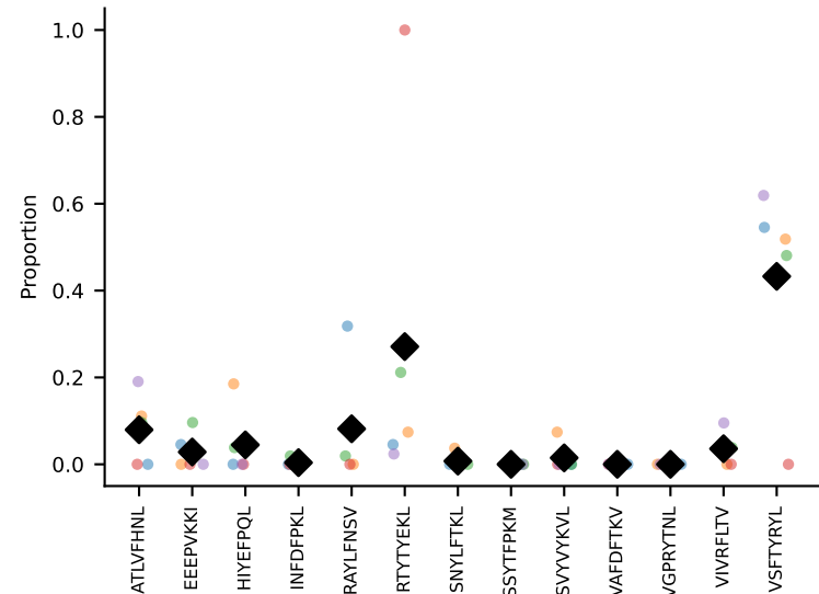
#5 AV10N-CAASMDTGGLSGKLTf-AJ2_BV16-CASSLNWGANAYAEQFF-BJ2-1 coh=0.386, n=13
