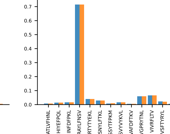
AV2-CIVTDSYSNNRLTL-AJ7_BV1-CTCSAGRGD AEQFF-BJ2-1 PROP n:36→35
