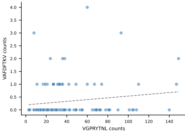
VAFDFTKV r=0.146 , p=1.18e-01
