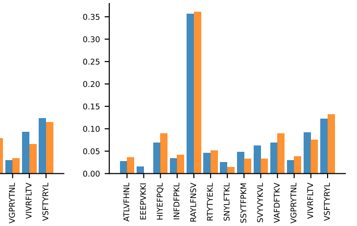
AV7-2-CAATGNTGKLIF-AJ37_BV19-CASSIRIAEQFF-BJ2-1 PROP n:9→8
