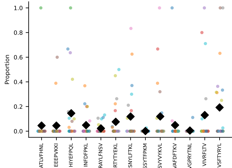
#80 AV13-2-CAIVPGTGSNRLTF-AJ28_BV3-CASSLSNTEVFF-BJ1-1 coh=0.178, n=8
