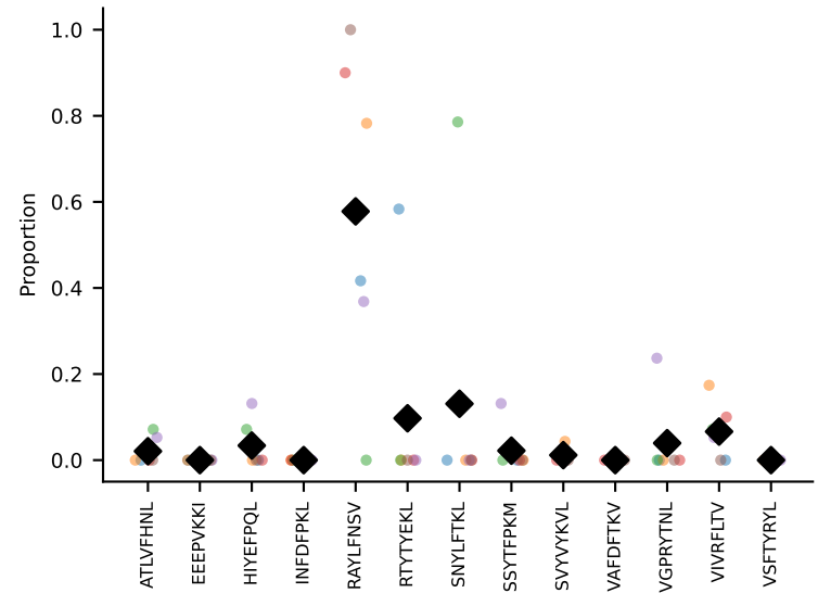
#20 AV7-2-CAATGNTGKLIF-AJ37_BV19-CASSIRIAEQFF-BJ2-1 coh=0.465, n=8
