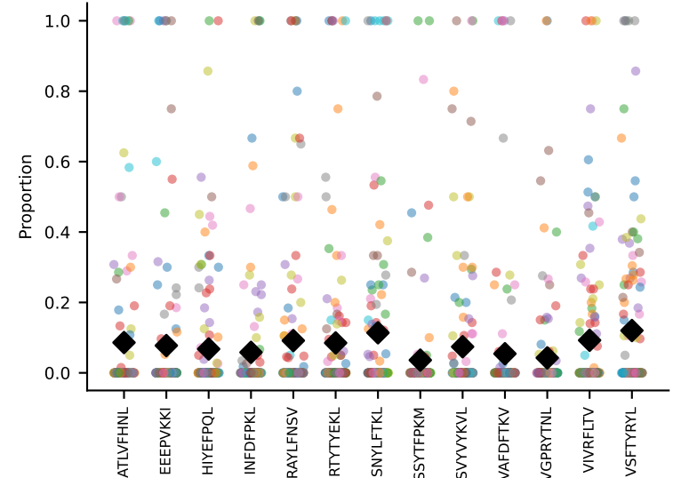
#104 AV12-2-CALNQGGSAKLIF-AJ57_BV1-CTCSADWGNYAEQFF-BJ2-2 coh=0.155, n=8
