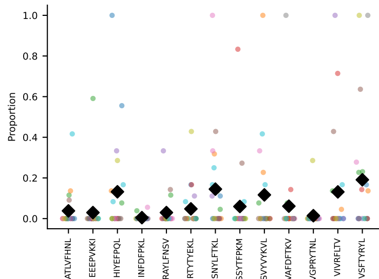
#119 AV7D-5-CAVKGQGTGSKLSF-AJ58_BV1-CTCSATGGGNQAPLF-BJ1-5 coh=0.217, n=20
