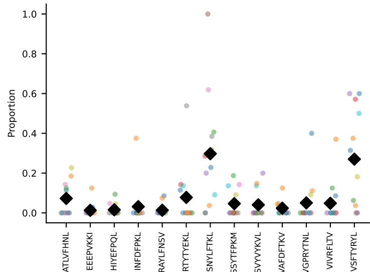
#23 AV13-1-CALEPSGSWQLIF-AJ22_BV1-CTCSAGTGGDTGQLYF-BJ2-2 coh=0.453, n=12
