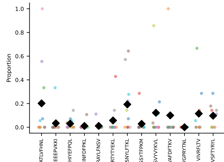
#125 AV3-3-CAVSAWANYNVLYF-AJ21_BV3-CASSLGRSYEQYF-BJ2-7 coh=0.207, n=77
