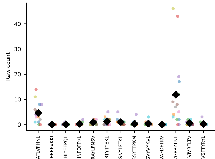
#288 AV8N-2-CATDSRGGRALIF-AJ15_BV3-CASSAGLGAEQYF-BJ2-7 coh=0.665, n=16
