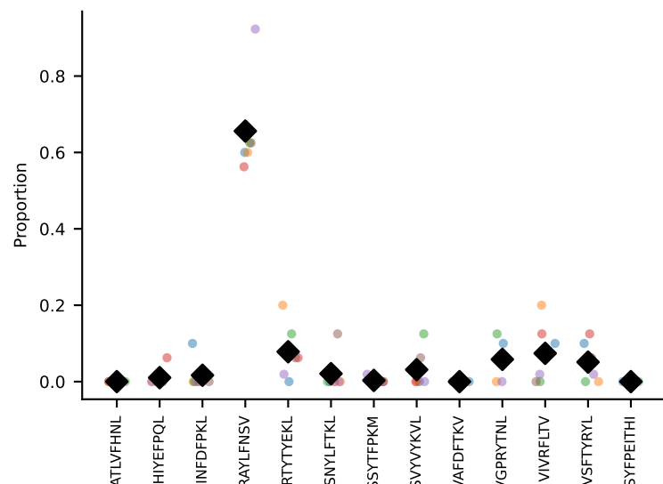
#155 AV12-2-CALTGGNNKLTF-AJ56_BV1-CTCSAGTGVGAETLYF-BJ2-3 coh=0.933, n=8
