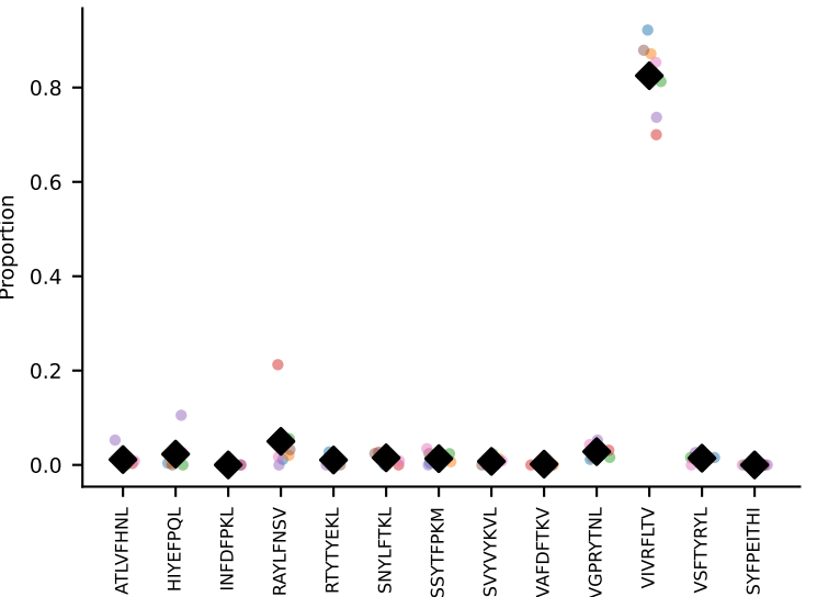
#91 AV2-CIVTDSYSNNRRTL-AJ7_BV1-CTCSAGRGD AEQFF-BJ2-1 coh=0.983, n=18
