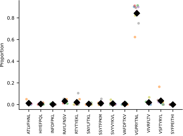
#70 AV5-1-CSASTDNNRIFF-AJ31_BV3-CASSYGTGGHEQYF-BJ2-7 coh=0.989, n=9
