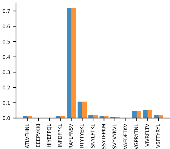
AV3D-3-CAVSGGNYKYF-AJ40_BV13-2-CASGDAGGATEQFF-BJ2-1 PROP n:6→6
