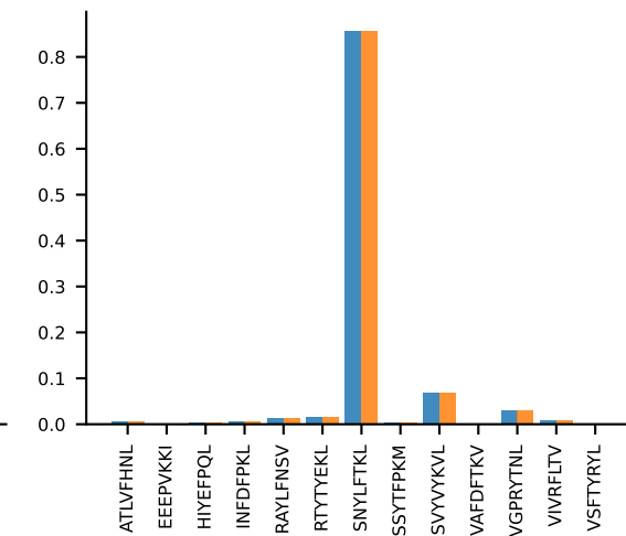
AV6-6-CALGENTNTGKLT-AJ27_BV2-CASSQDRRGDTQYF-BJ2-5 PROP n:5→5
