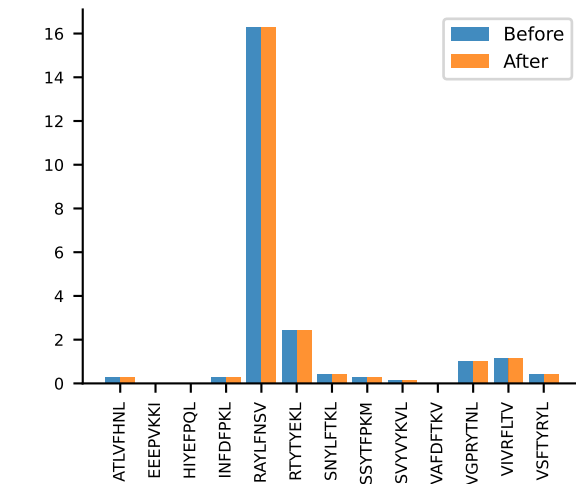
AV3D-3-CAVSGGNYKYF-AJ40_BV13-2-CASGDAGGATEQFF-BJ2-1 MEAN n:6→6
