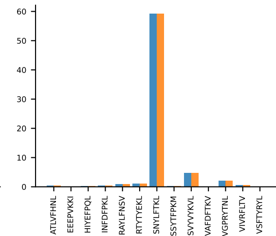
AV6-6-CALGENTNTGKLT-AJ27_BV2-CASSQDRRGDTQYF-BJ2-5 MEAN n:5→5
