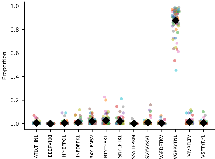
#33 AV13-2-CAIDPNTGKLT-F-AJ27_BV13-3-CASSETGPEVFF-BJ1-1 coh=0.981, n=5
