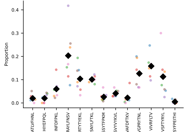
#116 AV16/DV11-CAMREGLGGNNKLTf-AJ56_BV1-CTCSAAGTGNTevff-BJ1-3 coh=0.781, n=5
