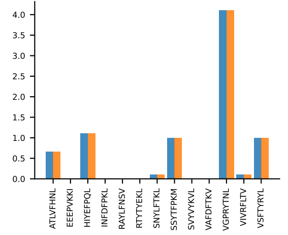
AV9-2-CVLSGDQGGRALIF-AJ15_BV3-CASSFSYEQYf-BJ2-7 MEAN n:9→9
