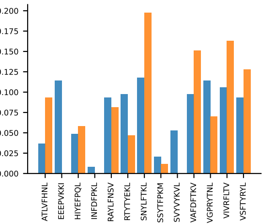
AV7-2-CAATGNTGKLIF-AJ37_BV19-CASSIRIAEQFF-BJ2-1 PROP n:9→8
