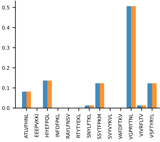
AV9-2-CVLSGDQGGRALIF-AJ15_BV3-CASSFSYEQYf-BJ2-7 PROP n:9→9
