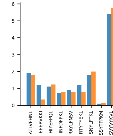
AV9-2-CVLSGDQGGRALIF-AJ15_BV3-CASSFSYEQYf-BJ2-7 MEAN n:9→9
