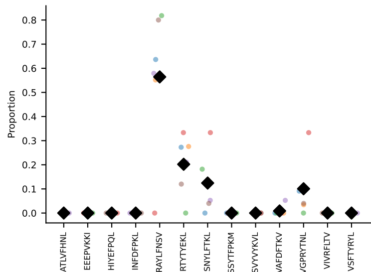
#361 AV6D-7-CALGRPGTGSNRLTF-AJ28_BV5-CASSQVAGDTEVFF-BJ1-1 coh=0.699, n=7
