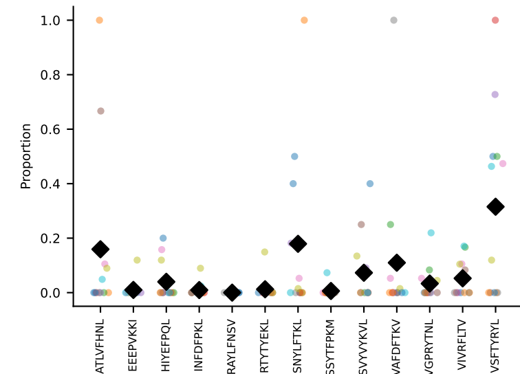
#53 AV3D-3-CAAGTGGYKVVF-AJ12_BV26-CASSLGLSNQDTQYF-BJ2-5 coh=0.311, n=8
