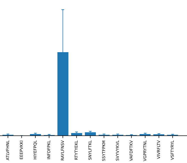
AV13-1-CALEMLYANKMIF-AJ47_BV13-2-CASGDYWGGAQFF-BJ2-1 (n=8)
