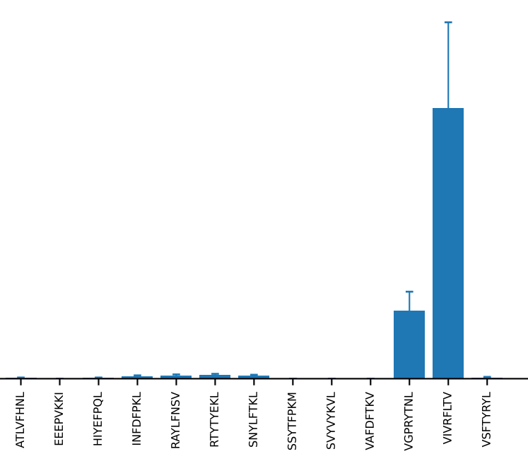
AV14-2-CAAIDSNRIFF-AJ31_BV13-3-CASSGGHLNTEVFF-BJ1-1 (n=8)
