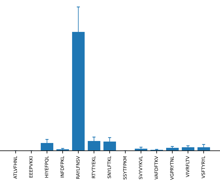
AV16/DV11-CAMRESNTGYQNFYF-AJ49_BV13-2-CASGEGQKNLTLYF-BJ2-4 (n=8)
