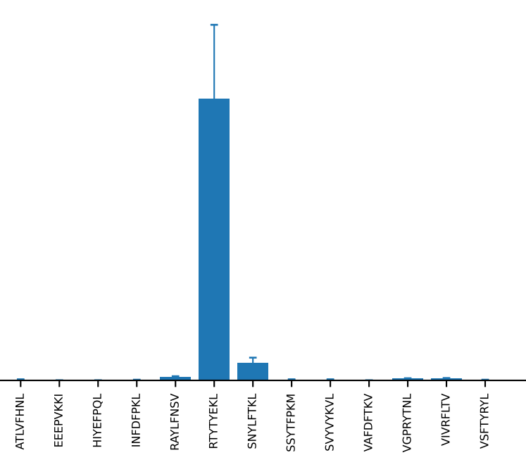
AV13-2-CAIDPNTGKLTf-AJ27_BV13-3-CASSDSNQAPLF-BJ1-5 (n=8)
