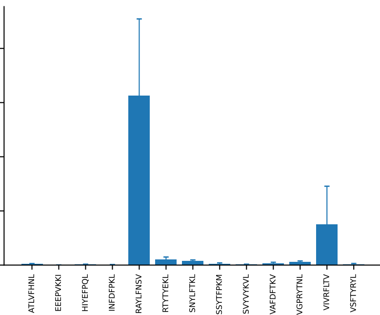
AV16-CAMREANYGNEKITF-AJ48_BV31-CAWSLRDINERLFF-BJ1-4 (n=10)
