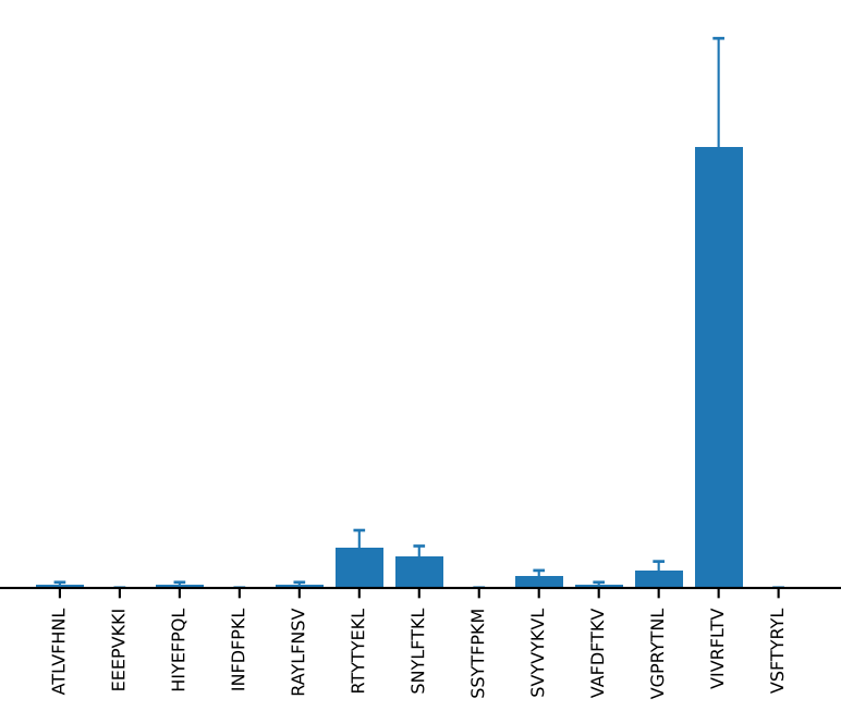
AV16/DV11-CAMREGDSNYQLIW-AJ33_BV13-2-CASGDRAANSDYTF-BJ1-2 (n=8)
