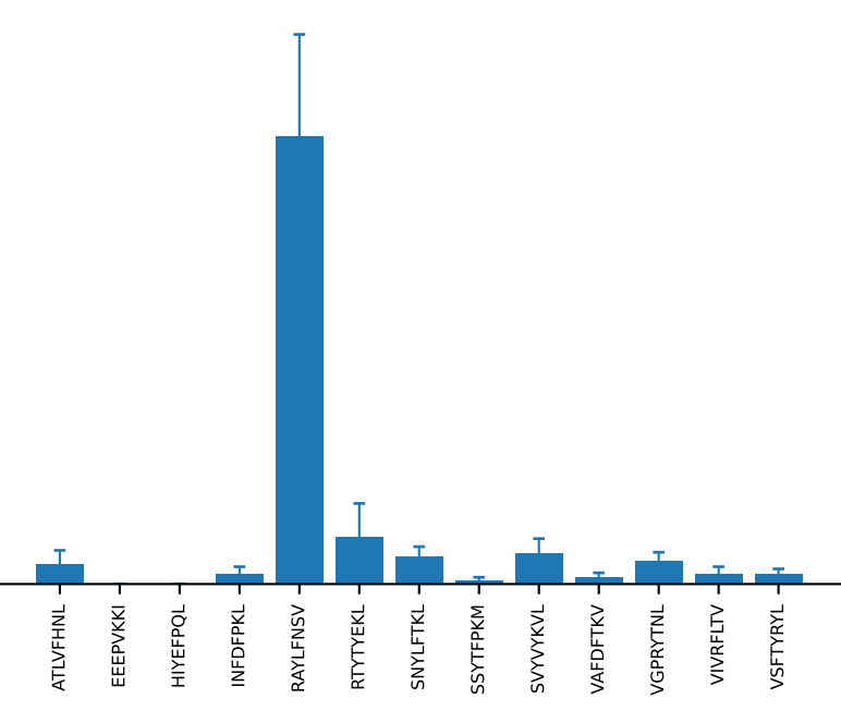
AV8D-2-CATDTGKLTf-AJ27_BV3-CASSLDSNERLFF-BJ1-4 (n=8)
