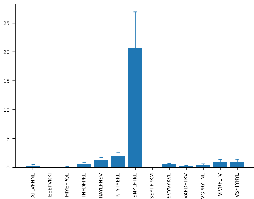
AV8-1-CATDGASSSFSLVF-AJ50_BV1-CTCSADGYEQYF-BJ2-7 (n=10)
