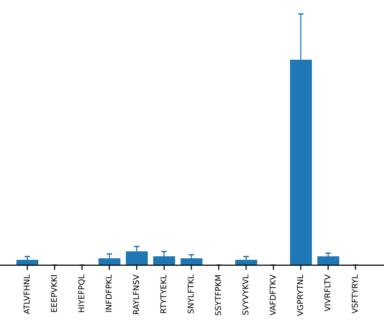
AV13N-3-CASNRIFF-AJ31_BV1-CTCSADRVTQYF-BJ2-5 (n=8)
