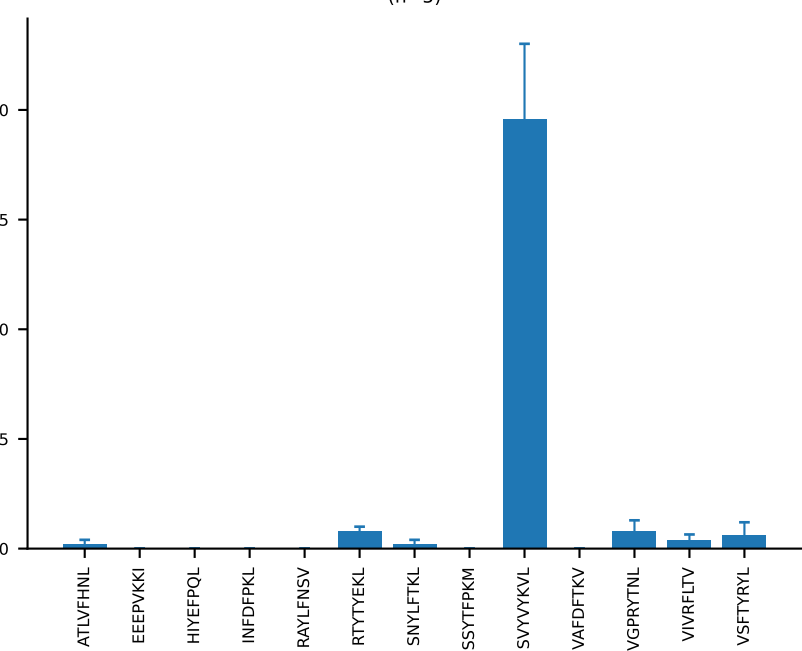
AV6-6-CALGENTNTGKLTIF-AJ27_BV2-CASSQDRRGDTQYF-BJ2-5 (n=5)
