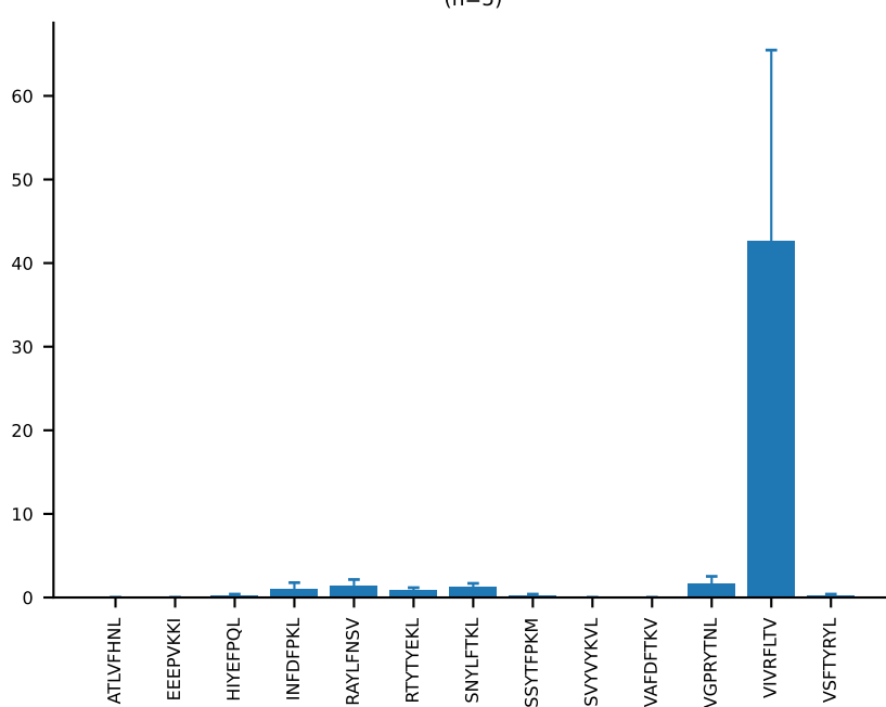
AV15-1/DV6-1-CALWELNNNAGAKLTIF-AJ39_BV3-CASSLGGGYEQYF-BJ2-7 (n=5)
