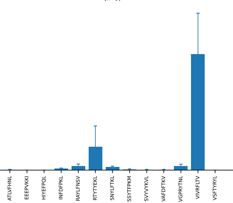
AV16N-CAMREDSNYQLIW-AJ33_BV16-CASSLDGLNYAEQFF-BJ2-1 (n=9)
