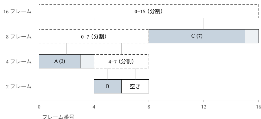
図 8.9: 例 8.20 のバディアロケーターの, ステップ 3 の後のブロック. 括弧内は要求されたフレーム数である. 破線のブロックは分割されており, 薄く塗ったフレームは内部断片化で失われている.
