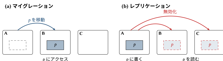
図 15.3: ページ p を、それにアクセスするノードのもとへ持ってくる。(a) マイグレーションは唯一のコピーを移動する。(b) レプリケーションは複数のノードに複製を保ち、それらは p をローカルに読む。所有者 A による書き込みは B と C の複製を無効化する (破線)。
