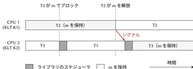
図 5.4: 2 つの CPU 上の、優先度が T3 > T2 > T1 であるユーザレベルスレッド。T2 が m をアンロックすると、CPU 1 のライブラリは K2 にシグナルを送り、CPU 2 のライブラリが T1 をプリエンプトして T3 を実行する。
