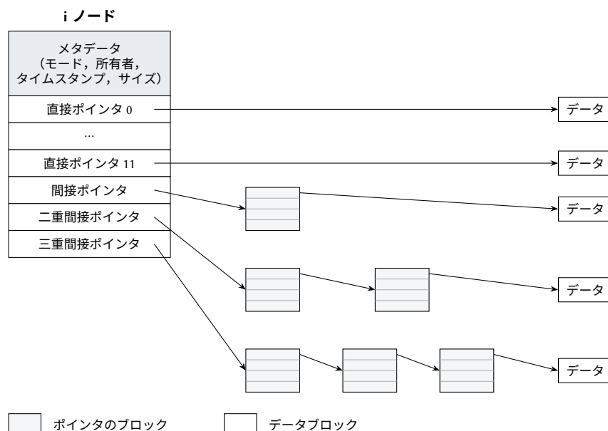
図 11.10: 12 個の直接ポインタと、単一・二重・三重の間接ポインタを持つ i ノード。間接の段が 1 つ増えるごとに、到達できるデータブロックの数は 1 ブロックあたりのポインタ数倍になる。
