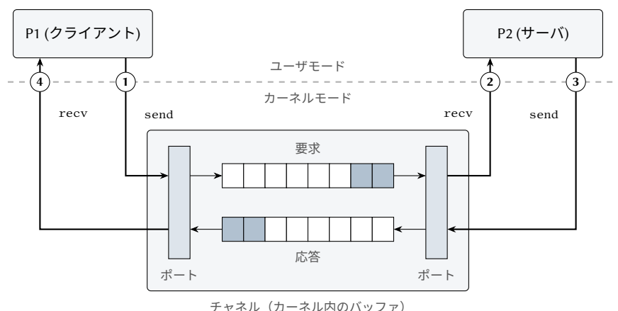
図 9.1: メッセージベースの IPC による要求・応答のやり取り。番号を付したユーザ/カーネル境界の横断はそれぞれ、1 回のシステムコールと、プロセスのアドレス空間とカーネルのチャンネルとの間の 1 回のコピーである。
