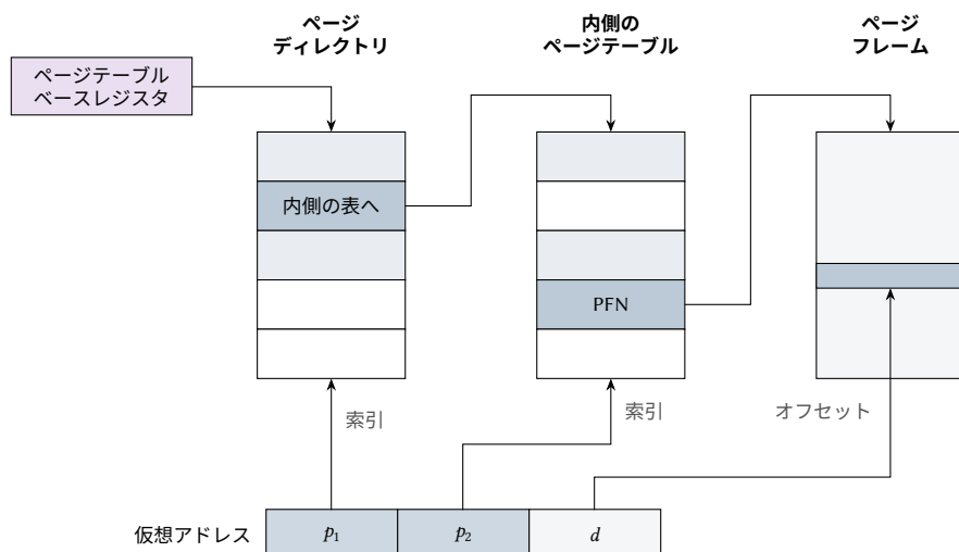
図 8.5: 2 段のページテーブル。白いディレクトリエントリには内側のページテーブルがない。変換には、ページディレクトリへの 1 回と内側のページテーブルへの 1 回のアクセスを要する。
