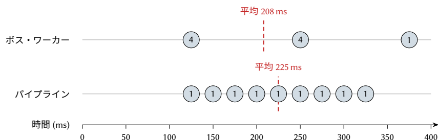
図 6.1: 9 個の要求の完了時刻. 各円はその時刻に完了する要求の数を示す. 4 つのワーカーを持つボス・ワーカーは 125 ms ごとに 4 個の要求を完了し, 5 段のパイプラインは最初の 125 ms の後は 25 ms ごとに 1 個の要求を完了する. 破線は平均完了時間を示す.
