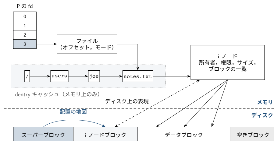
図 11.8: VFS の抽象化。プロセス P のファイルディスクリプタ 3 は開いたファイルを指し、そのファイルの dentry が i ノードへ導く。パスの dentry はメモリ上にのみ存在する。ディスク上では、スーパーブロックが i ノード・データ・空き領域を保持するブロックの地図となる。
