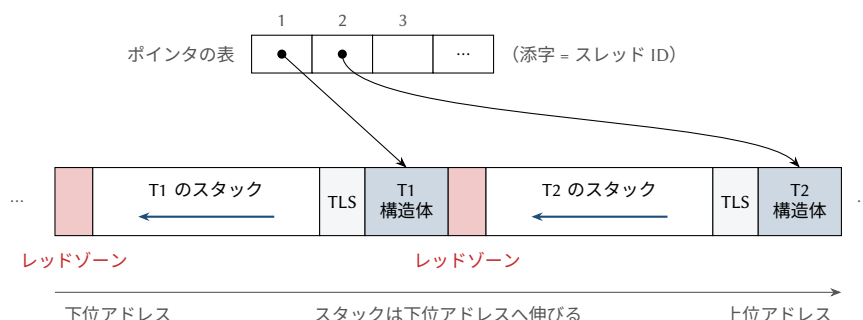
図 5.3: 連続して割り当てられたユーザレベルスレッドのデータ構造。スレッド識別子は、構造へのポインタの表への添字である。T2 のスタックがあふれても、T1 の構造に達する前にレッドゾーンに入る。
