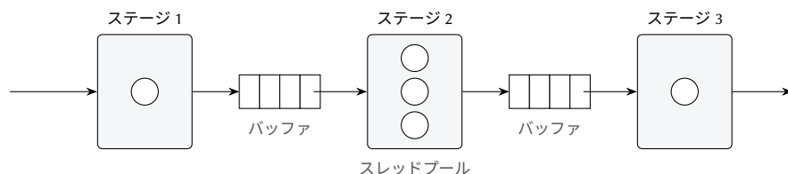
図 3.8: 3 ステージのパイプライン。ステージはバッファを通じて要求を受け渡す。遅い第 2 ステージは 3 スレッドのプールである。
