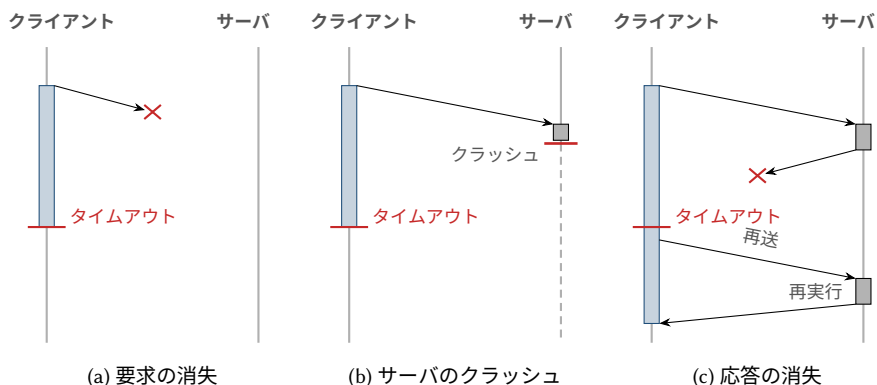
図 13.3: クライアントが区別できない 3 つの部分障害。網掛けの帯はクライアントがブロックしている時間を、灰色の箱は手続きの実行を、× は失われたメッセージを表す。(a) 要求が失われる。(b) 呼び出しの実行中にサーバがクラッシュする。(c) 応答が失われ、再送が手続きを 2 度目に実行する。
