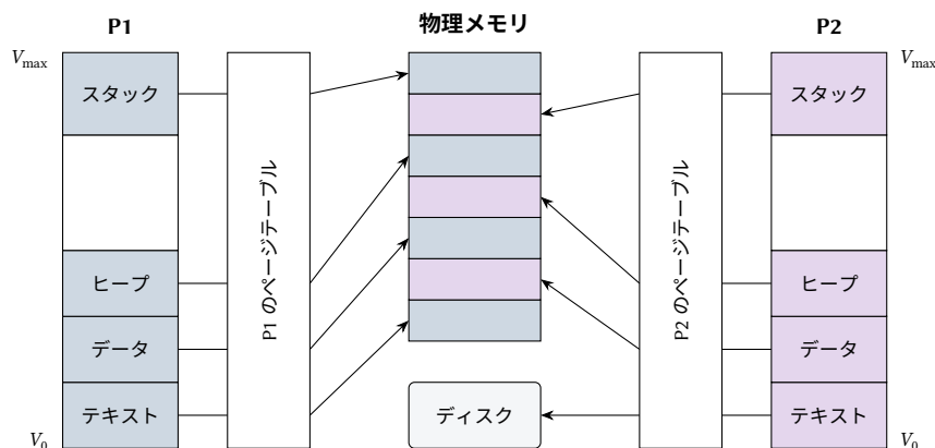
図2.2: 同じ仮想アドレスの範囲を持つ2つのプロセス。それぞれのページテーブルは、割り当てられた領域を異なる物理フレームへ対応付けている。P2のテキストは現在ディスク上にあり、割り当てられていない領域はどこにも対応付けられていない。
