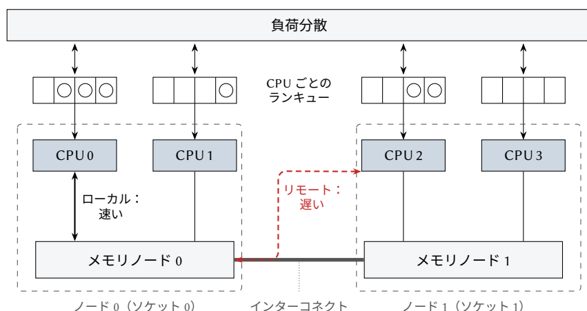
図 7.9: NUMA システム上の階層的なスケジューリング。どの CPU も自分のランキューからタスクをスケジューリングし、負荷分散がランキューの間でタスクを移動させる。CPU は自分のノードのメモリには直接、もう一方のノードのメモリにはインターコネクトを経由して到達する。
