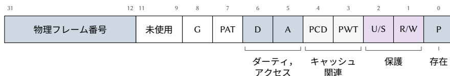
図 8.4: 32 ビット x86 のページテーブルエントリ。グローバルビット G とページ属性ビット PAT はここでは扱わない。
