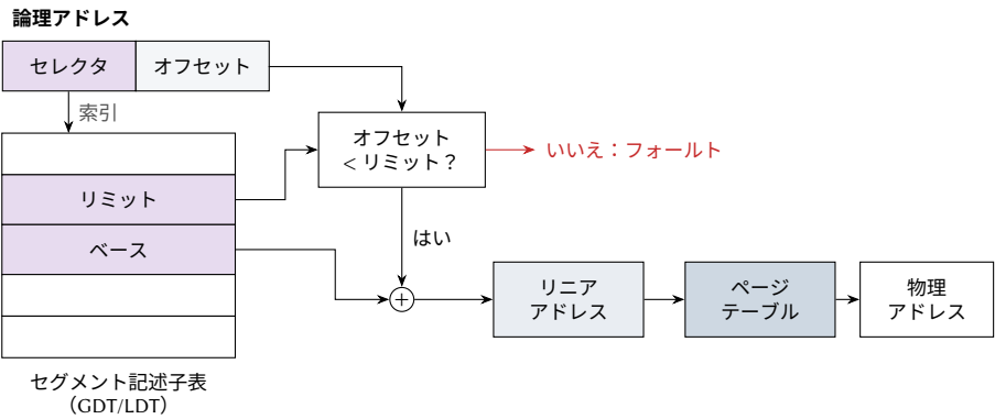
図 8.7: x86 における、ページングと組み合わせられたセグメンテーション。セクタがセグメント記述子表の索引となる。リミット内のオフセットがベースに加えられ、得られたリニアアドレスがページテーブルによって変換される。
