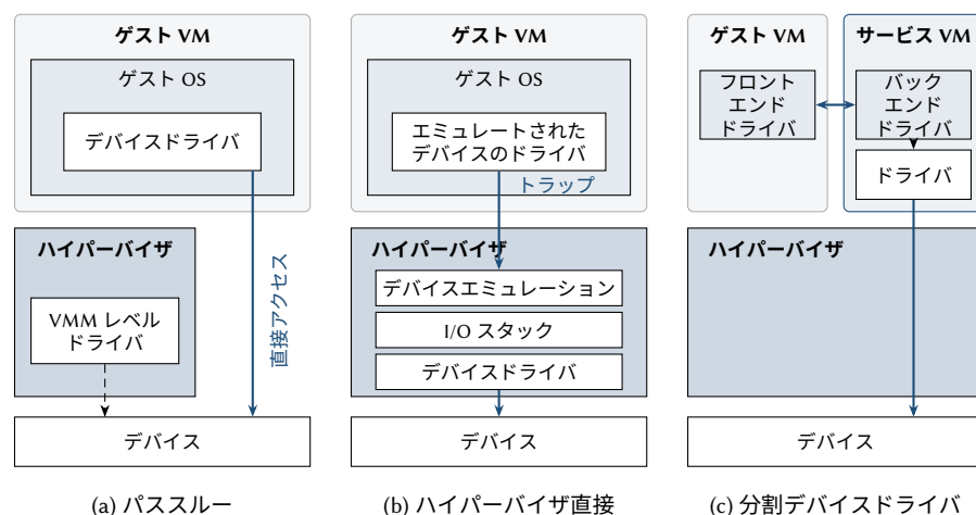
図 12.7: デバイスの仮想化のモデル。(a) VM 自身のドライバがデバイスに直接アクセスする。(b) ハイパーバイザがデバイスアクセスを横取りし、自分の I/O スタックとドライバでそれをエミュレートする。(c) ゲスト内のフロントエンドドライバが、サービス VM 内のバックエンドドライバに要求を渡し、バックエンドドライバがデバイスを駆動する。
