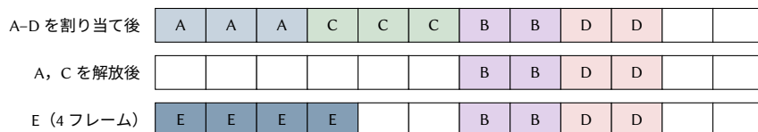
図 8.8: 12 フレームのプールにおける外部断片化. 同じ要求と解放の並びが, アロケーターが A と C をどこに配置したかに応じて, (a) 3 つの小さな穴を残すか, (b) 1 つの大きな穴を残す.
