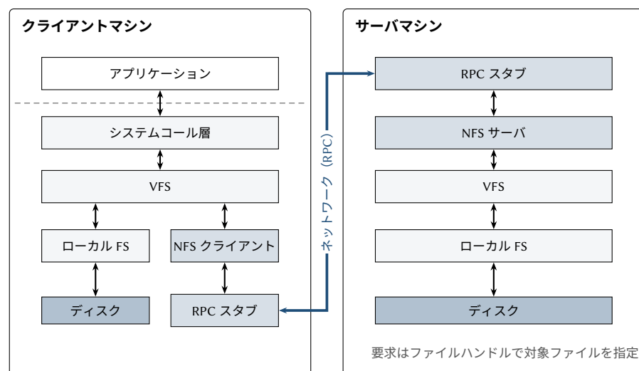
図 14.6: NFS. クライアントの VFS は NFS ファイルに対する操作を NFS クライアントへ渡し、NFS クライアントはそれを RPC 要求として NFS サーバへ送る。サーバは自身の VFS とローカルファイルシステムを通じてそれを実行する。
