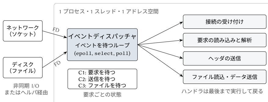
図 6.4: イベント駆動のウェブサーバ。ディスパッチャはファイルディスクリプタ（FD）上のイベント—準備の整ったソケット、および非同期 I/O やヘルパ（6.6 節）が完了を通知するディスク読み込み—を待ち、イベントごとにそのハンドラを呼び出す。処理中の各要求の状態は、明示的なレコードに保持される。
