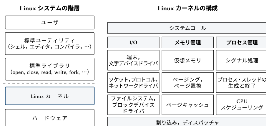
図 1.5: 左: Linux システムの階層. 破線はユーザ/カーネル境界である. 右: Linux カーネルの構成要素 (Tanenbaum と Bos [5] による).
