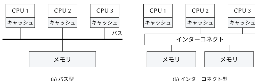
図 10.4: 共有メモリ型マルチプロセッサの構成。どちらでも、各 CPU が自分のキャッシュを持ち、すべての CPU がすべてのメモリにアクセスできる。
