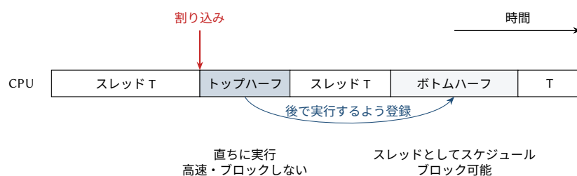
図 5.6: トップハーフとボトムハーフに分けた割り込み処理。トップハーフはスレッド T に割り込み、ボトムハーフはスケジューラが後で実行する。
