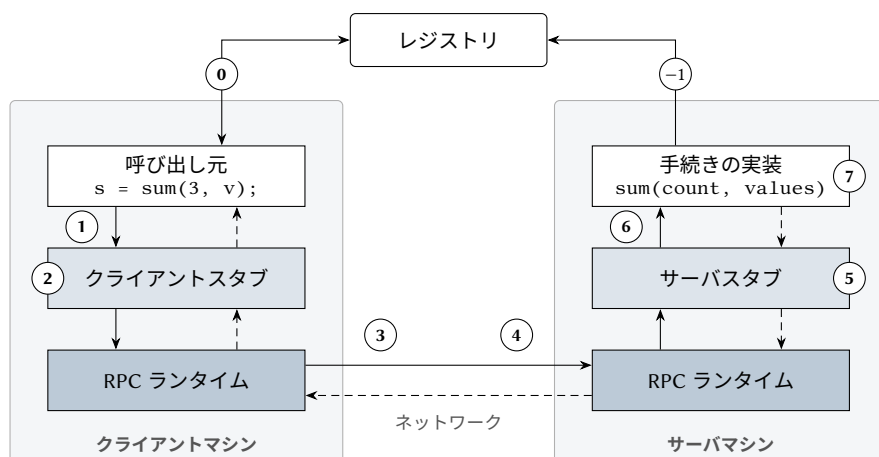
図 13.1: RPC システムの構造と呼び出しの手順。実線の矢印は呼び出しを、破線の矢印は結果の返送を表す。手順 -1 と 0 は最初の呼び出しの前に行われる。
