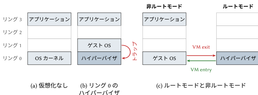
図 12.3: x86 の保護リングの使い方。 (a) 仮想化なしの実行。 (b) ハードウェア支援のない仮想化: ゲスト OS はリング 1 へ降格され、その特権的な操作はハイパーバイザへトラップする。 (c) 仮想化支援を備えたプロセッサ: ゲスト OS は非ルートモードのリング 0 で動作し、VM exit が制御をルートモードのハイパーバイザへ移す。
