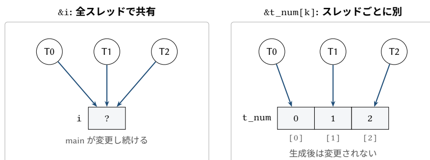
図 4.2: 左: すべてのスレッドがループ変数 i のアドレスを受け取り、その値はスレッドの起動中に変化する。右: 各スレッドは自分専用の配列要素のアドレスを受け取り、その値はスレッドの生成後に変化しない。
