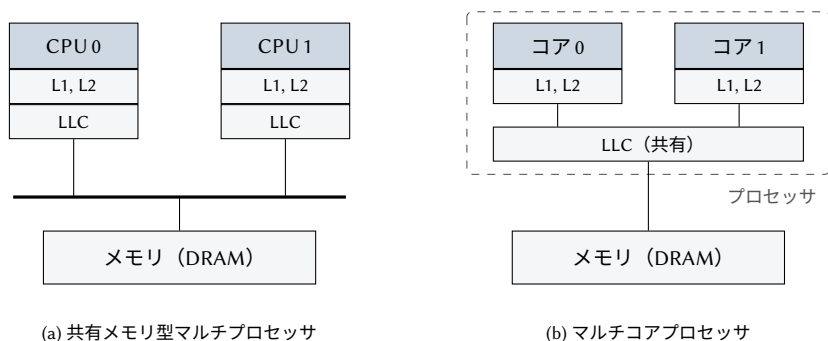
図 7.8: (a) 共有メモリ型マルチプロセッサ. どの CPU も自分専用のキャッシュを持つ. (b) マルチコアプロセッサ. コアは専用のキャッシュを持ち, ラストレベルキャッシュを共有する.
