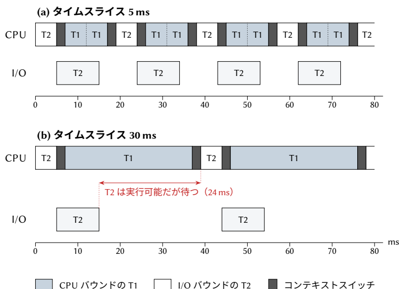
図 7.4: ラウンドロビンの下での CPU バウンドのタスク T1 と I/O バウンドのタスク T2 (例 7.16)。T2 がまだ I/O を待っている間に T1 のタイムスライスが満了した場合、T1 はそのまま実行を続ける。
