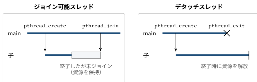
図 4.1: 左: ジョインされる前に終了したジョイン可能な子は, pthread_join がステータスを回収するまで資源を保持する。右: デタッチされた子は自分で資源を解放する。メインスレッドは pthread_exit で終了し, 残りのスレッドがジョイン可能かデタッチされているかによらずプロセスは動き続ける。
