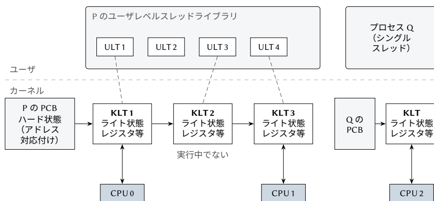
図 5.1: 大規模な場合のスレッドのデータ構造。プロセスの PCB は、そのすべてのスレッドが共有する状態と、カーネルレベルスレッド (KLT) のリストを保持する。各 KLT は独自の状態を保持し、実行中は CPU に結び付けられる。破線は、ライブラリが現在のユーザレベルスレッド (ULT) をどの KLT に配置しているかを示す。KLT から PCB への逆向きのポインタは省いてある。
