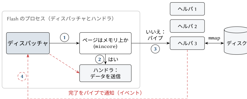
図 6.5: Flash におけるファイルデータの提供. (1) ディスパッチャが mincore でデータがメモリ上にあるかを調べる. (2) あれば, ハンドラが直接を送る. (3) なければ, ヘルパにパイプでページへのアクセスを依頼し, ヘルパがディスクから読み込む. (4) その完了報告がイベントとなり, その後ハンドラがデータを送る.
