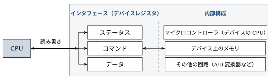
図 11.1: 基本的な I/O デバイス。CPU はコマンド・ステータス・データの各レジスタを通じてのみデバイスとやり取りする。コマンドを実行する内部構成はデバイス固有である。
