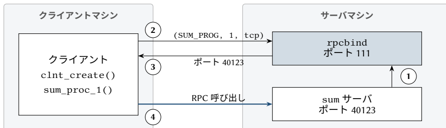
図 13.5: Sun RPC における登録とバインディング。(1) サーバが自分のプログラム、バージョン、トランスポート、ポートを rpcbind に登録する。(2,3) clnt_create がサーバマシンの rpcbind にポートを尋ねる。(4) 呼び出しは直接サーバへ送られる。
