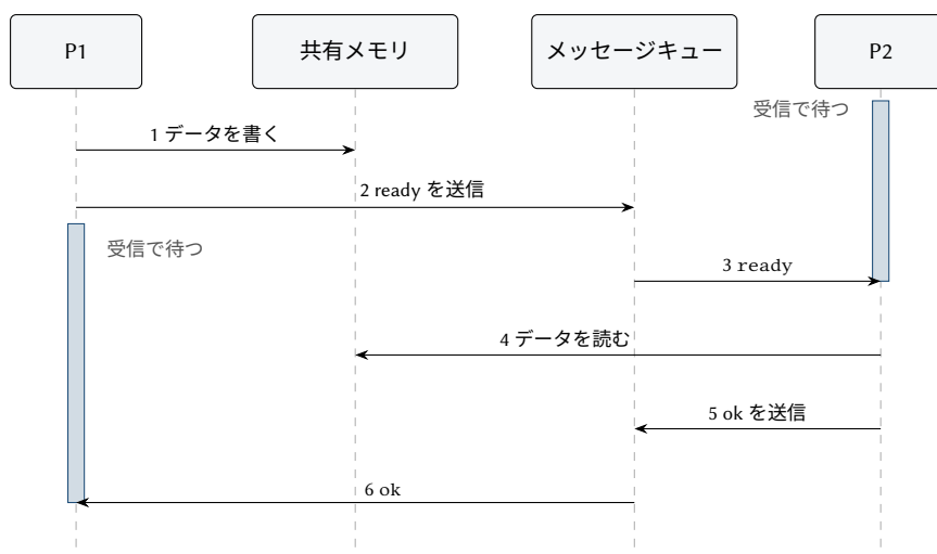
図 9.4: メッセージキューが共有メモリへのアクセスを協調させる。P2 は「ready」の後のみ読み、P1 は「ok」の後のみ先へ進む。
