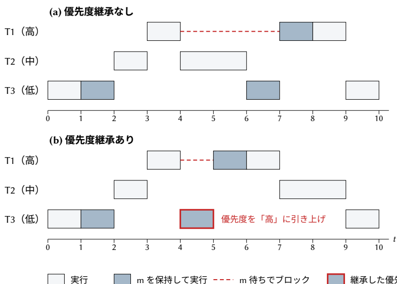
図 7.3: T1 と T3 はミューテックス m を共有する。(a) T1 が m でブロックしている間に、中優先度の T2 が T1 に先んじて完了まで実行される。(b) 優先度継承があると、 T3 は m をアンロックするまで T1 の優先度で実行され、 T1 は T2 より先に完了する。
