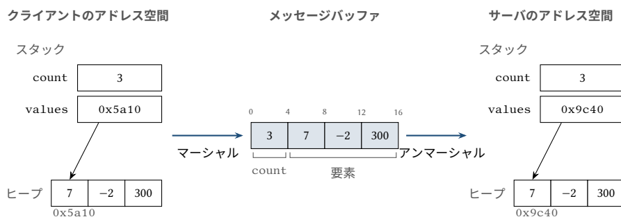
図 13.2: sum(3, v) の引数のマーシャリングとアンマーシャリング。バッファには、ポインタが指す配列を含めて引数の値が入るが、ポインタそのものは入らない。その上に付した数はバイトオフセットである。
