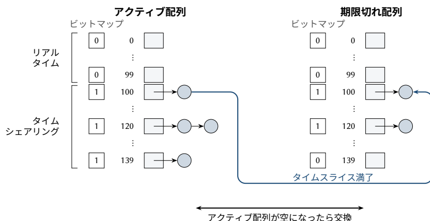
図 7.6: O(1) スケジューラのランキュー。各配列は優先度の水準ごとに 1 本のリストと、空でないリストを示すビットマップを持つ。タイムスライスが満了したタスクは期限切れ配列へ移り、アクティブ配列が空になると 2 つの配列が交換される。
