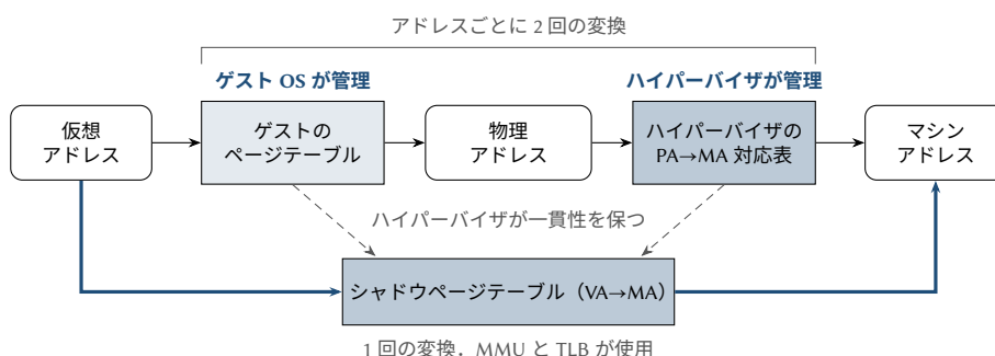
図 12.6: メモリの仮想化。ゲストのページテーブルを通り、次にハイパーバイザの対応表を通る変換は 2 段階を要する。シャドウページテーブルは両者を、MMU が直接使う 1 つの対応にまとめる。拡張ページテーブルを備えたハードウェアは、この 2 段階の変換を自ら行う (12.11 節)。
