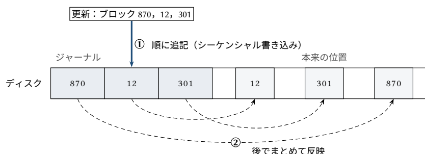
図 11.11: ジャーナリング。散らばったブロックへの更新は、まず順にジャーナルへ追記され、後から本来の位置へ反映される。
