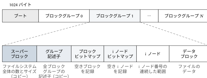
図 11.9: ext2 のパーティションの配置。ブート用に予約された領域の後、パーティションはブロックグループに分割され、各グループはスーパーブロックとグループ記述子表のコピー、自身のビットマップ、そして i ノードとデータブロックを持つ。
