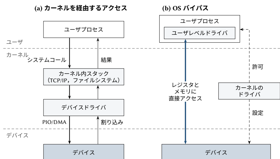
図 11.4: (a) 典型的なデバイスアクセスは、システムコール、カーネル内スタック、デバイスドライバを通る。(b) OS バイパスでは、プロセスはユーザーレベルドライバを通じてデバイスにアクセスし、カーネルはアクセスの設定と制御を行うだけである。
