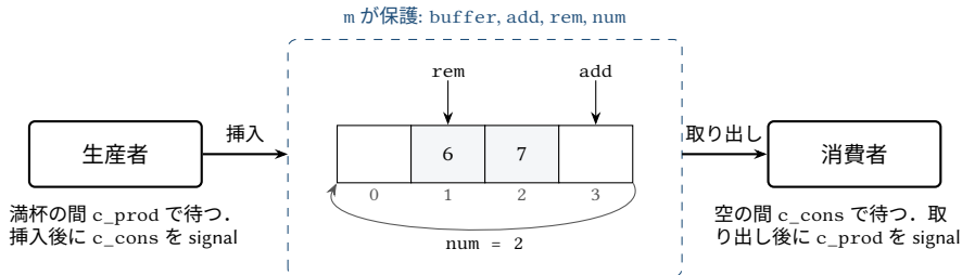
図 4.3: BUF_SIZE = 4 の生産者・消費者プログラム. 1 つのミューテックスがバッファの状態をすべて保護し, 各スレッドは自分専用の条件変数で待つ.
