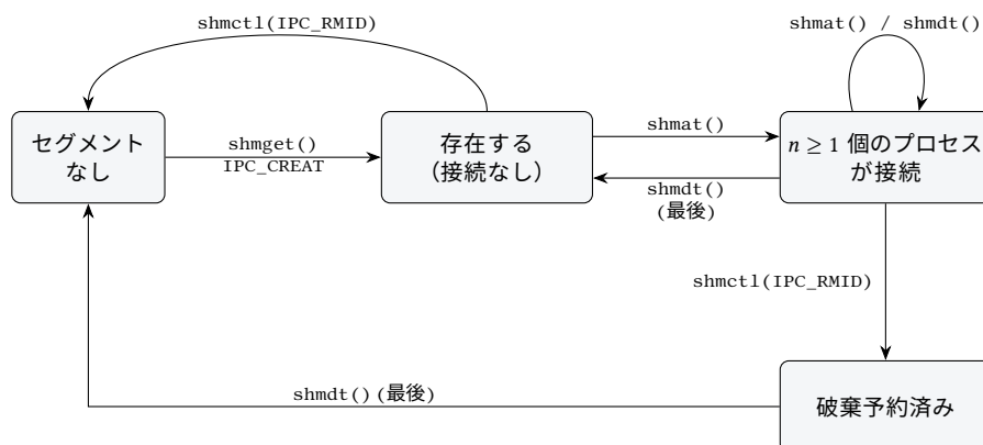
図 9.3: System V 共有メモリセグメントのライフサイクル。セグメントはそれを使うプロセスより長く残り、取り除かれるのは IPC_RMID によってのみである。接続されたまま取り除かれたセグメントは、最後のプロセスが切り離した時点で破棄される。
