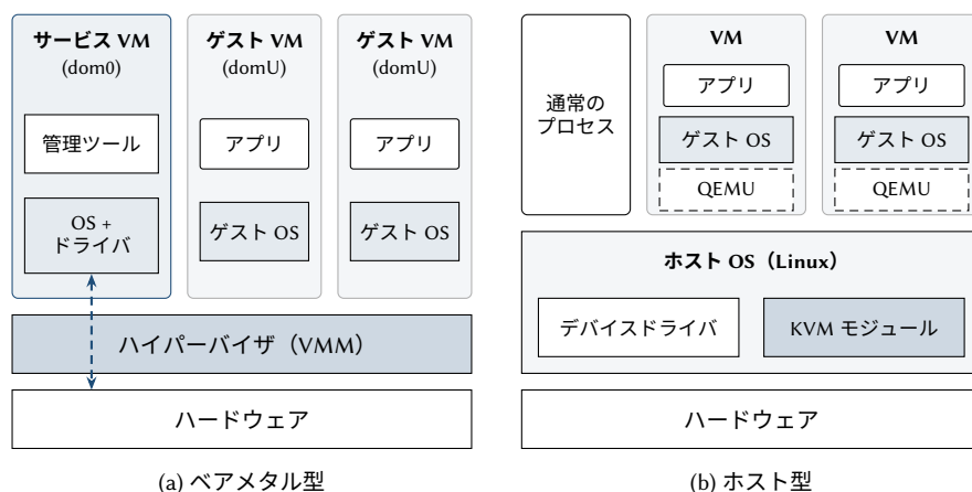
図 12.2: 仮想化のモデル。 (a) デバイスドライバを所有する特権的なサービス VM を伴うベアメタル型ハイパーバイザ。Xen がこの形である。 (b) ホスト型ハイパーバイザ: Linux における KVM のようにホスト OS のモジュールであり、各 VM はホストのプロセスで、その中で QEMU がデバイスをエミュレートする。
