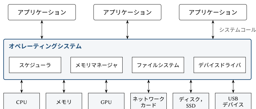
図 1.1: アプリケーションとハードウェアの間のオペレーティングシステム。アプリケーションはシステムコールを通じてサービスを要求し、スケジューラ、メモリマネージャ、ファイルシステム、デバイスドライバなどの構成要素がそれをハードウェア上で実行する。
