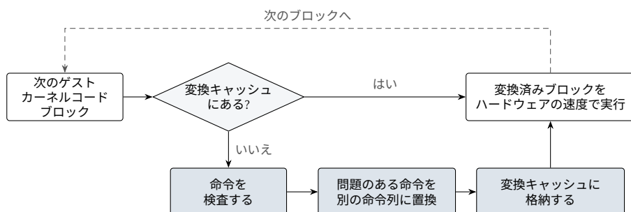
図 12.5: 変換キャッシュを伴う動的バイナリ変換。ブロックが検査され変換されるのは、最初に実行されようとするときだけである。
