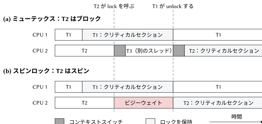
図 10.1: 別の CPU 上の T1 が保持するロックを T2 が要求する。(a) ミューテックスでは T2 はブロックし、CPU は別のスレッドを実行し、アンロックの後に T2 が戻される。(b) スピンロックでは T2 はビジーウェイトし、T1 がアンロックすると同時にクリティカルセクションに入る。
