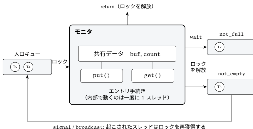
図 10.2: モニタ。スレッドはエントリ手続きを通じてのみ内部に入り、エントリ手続きはモニタのロックを暗黙的に獲得する。条件変数上で待つスレッドはロックを解放し、ここで示した Mesa のセマンティクスでは、起こされた後にロックを再獲得しなければならない。
