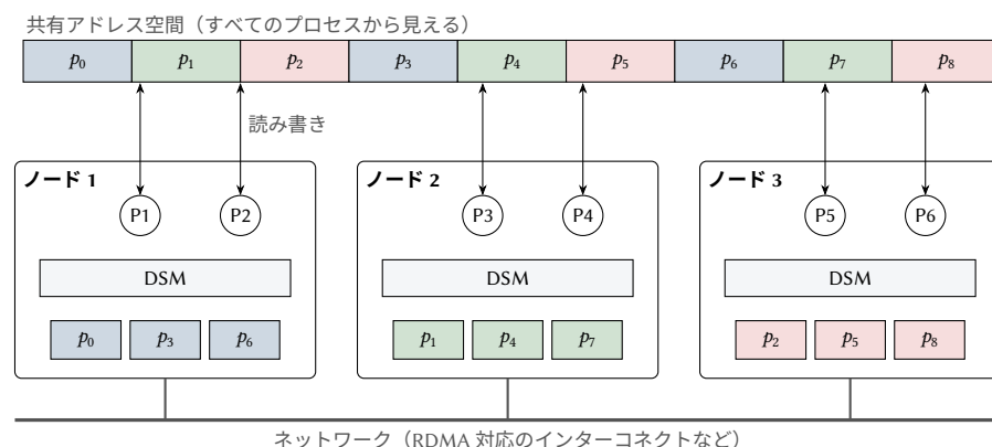
図 15.1: 分散共有メモリ。共有アドレス空間の各ページ p_i は、いずれかのノードが提供したメモリに存在する。各ノードの DSM 層は、ローカルなページへのアクセスを処理し、リモートのページをネットワーク越しに取得する。
