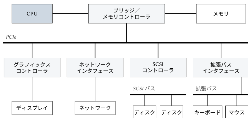
図 11.2: 典型的なプラットフォームのインターコネクト。デバイスコントローラは PCIe に接続され、ディスクとキーボードはそれぞれのコントローラの先の別のバスに接続される。PCIe は簡単のためバスとして描いてあるが、実際には各コントローラは自身のポイントツーポイントリンクで接続される。
