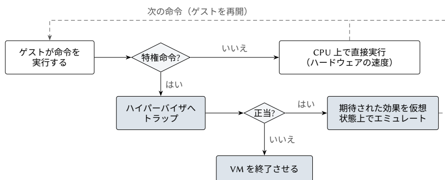
図 12.4: トラップアンドエミュレート。ハイパーバイザが関与するのは特権命令だけであり、正当なものは VM の仮想状態でエミュレートされる。
