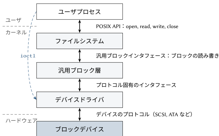
図 11.6: ブロックデバイススタック。各層は、その下に示したインタフェースを使う。ioctl はデバイス固有の要求をドライバへ運ぶ。
