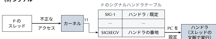
図 5.5: (a) デバイスが発生させた割り込みは, システム全体の割り込みハンドラテーブルからハンドラを選ぶ. (b) 不正なメモリアクセスによりカーネルが SIGSEGV を発生させ, これがプロセスのシグナルハンドラテーブルからハンドラを選ぶ.
