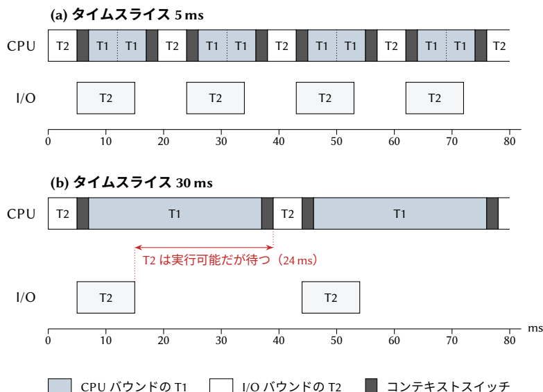
図 7.4: ラウンドロビンの下での CPU バウンドのタスク T1 と I/O バウンドのタスク T2 (例 7.16)。T2 がまだ I/O を待っている間に T1 のタイムスライスが満了した場合、T1 はそのまま実行を続ける。
