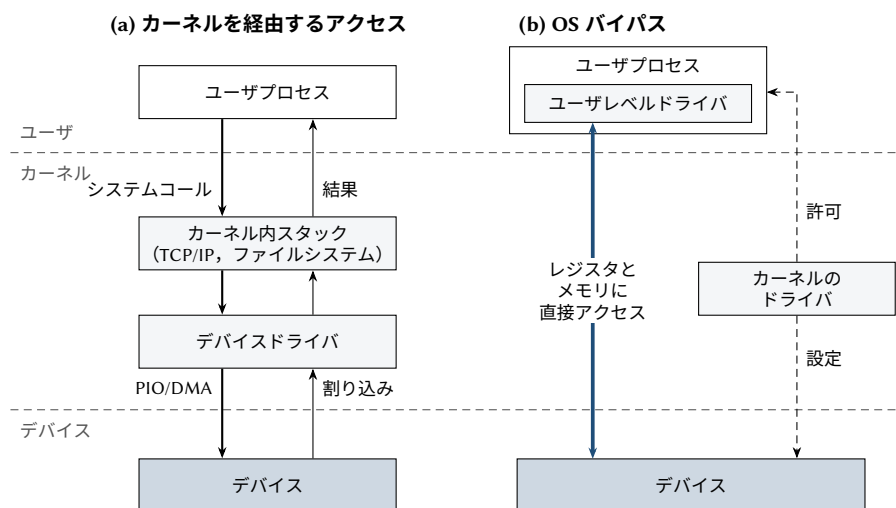
図 11.4: (a) 典型的なデバイスアクセスは、システムコール、カーネル内スタック、デバイスドライバを通る。(b) OS バイパスでは、プロセスはユーザレベルドライバを通じてデバイスにアクセスし、カーネルはアクセスの設定と制御を行うだけである。
