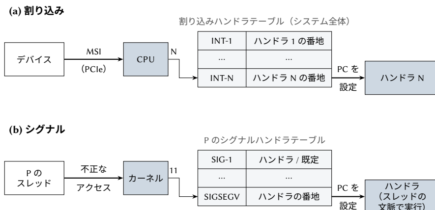
図 5.5: (a) デバイスが発生させた割り込みは, システム全体の割り込みハンドラテーブルからハンドラを選ぶ. (b) 不正なメモリアクセスによりカーネルが SIGSEGV を発生させ, これがプロセスのシグナルハンドラテーブルからハンドラを選ぶ.
