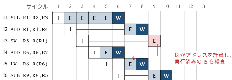
(b) ロードストアのインオーダー実行
