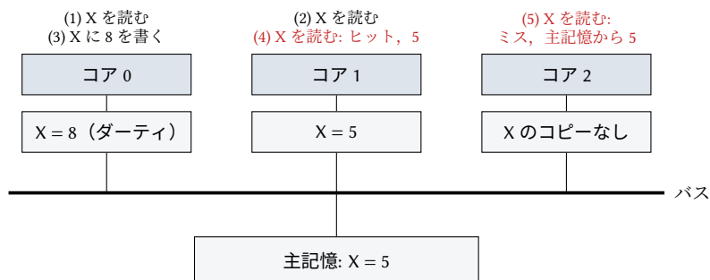
図 19.1: コヒーレントでないキャッシュ。コア 0 とコア 1 が、5 を保持する X を読み (手順 1 と 2)、コア 0 が自分のキャッシュに 8 を書く (手順 3)。その後のコア 1 の読み出し (手順 4) とコア 2 の読み出し (手順 5) は、どちらも古い値 5 を返す。
