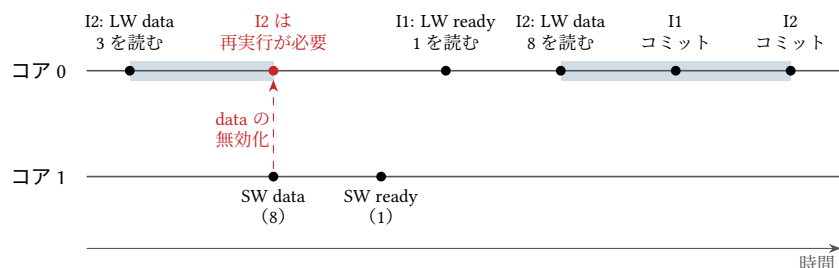
図 21.2: 順序変更されたロードの再実行。プログラム順では、コア 0 は I1: LW ready, 次に I2: LW data を実行する。I2 が実行済みでコミットしていない間 (網掛け) にコア 1 がデータを書き、その無効化によって I2 は再実行される。
