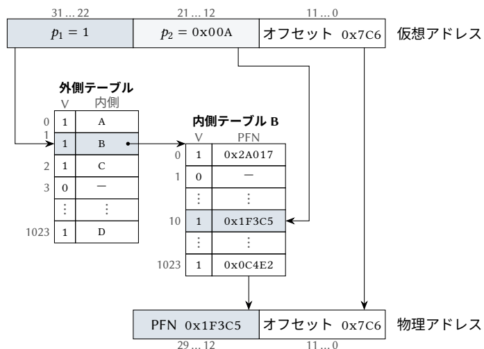
図 13.13: 仮想アドレス 0x0040A7C6 の 2 段の変換 (例 13.13)。外側のエントリ 1 は内側テーブル B を指す。A, C, D のエントリは図示していない内側テーブルを指す。エントリ 3 のような無効な外側エントリには、内側テーブルがそもそも存在しない。
