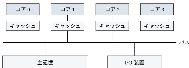
図 18.2: 集中共有メモリ: すべてのコアが同じバスを通じて主記憶と I/O 装置に到達する。
