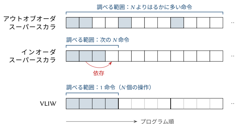
図 11.1: 1 サイクルを最大 N = 4 個の操作で埋めるために、各設計が調べる範囲。網掛けの箱がこのサイクルで実行される。インオーダの設計は、グループ内の先行する命令に依存する最初の命令で止まる。
