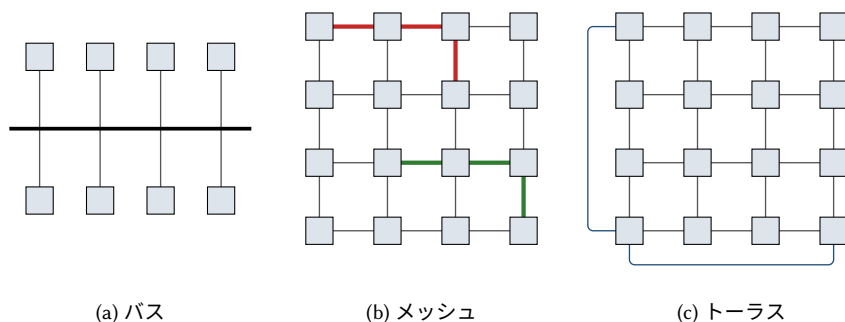
図 22.1: メニーコアのための相互接続網。バスは一度に 1 つの転送しか運ばない。メッシュは強調した 2 つの転送を異なるリンク上で同時に運ぶ。トーラスは各行各列の最初と最後のルータの間に折り返しリンクを加える—図では左端の列のものと最下行のものだけを描いている。
