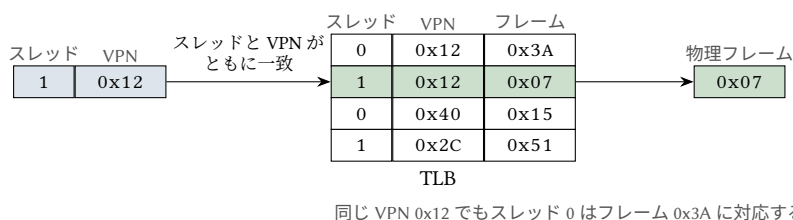
図 18.6: スレッドを意識した TLB。同じ仮想ページ番号が、2つのスレッドに対して別々のフレームに変換される。
