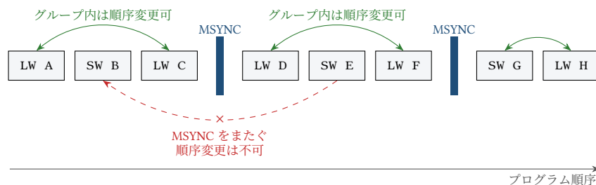
図 21.3: MSYNC は、コアのアクセスをプログラム順にグループへ分ける。1 つのグループ内の異なる位置へのアクセスは、モデルが許す範囲で異なる順序で効力を生じてよい。前のグループのアクセスより前に効力を生じるアクセスはない。
