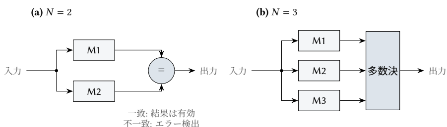
図 17.3: N モジュール冗長。 (a) 2 つのモジュールと比較器は、一方のモジュールにフォールトがあることは検出できるが、どちらであるかは分からない。 (b) 3 つのモジュールと多数決器は、いずれか 1 つのモジュールの誤った出力を隠蔽する。
