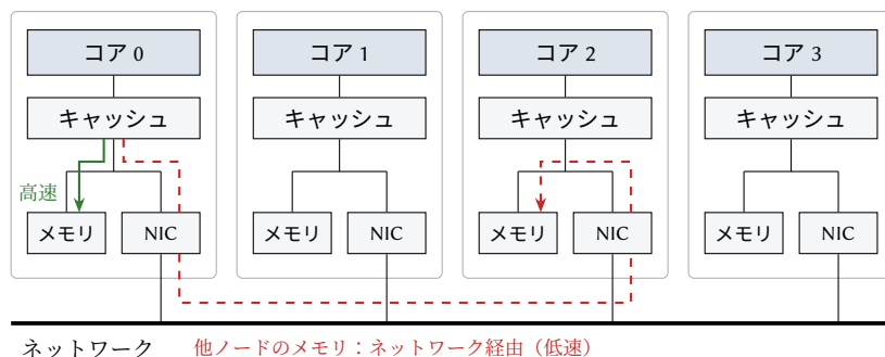
図 18.3: 分散共有メモリ: 各ノードは、コア、そのキャッシュ、ローカルメモリ、ネットワークインタフェースカード (NIC) からなる。
