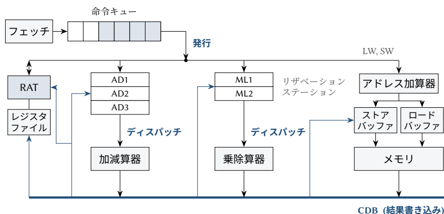
図 7.1: Tomasulo のアルゴリズムを用いるプロセッサの構成。発行は、RAT とレジスタファイルを用いて、キューの先頭の命令をリザベーションステーションに移す。ディスパッチは、準備のできた命令をその実行ユニットに送る。結果は共通データバスを通過して、リザベーションステーション、RAT、レジスタファイル、ストアバッファに戻る。ロードとストアは、アドレス加算器とロードバッファ・ストアバッファを経由する経路をとる。
