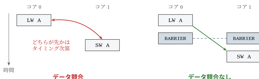
図 21.4: 左: A のロードとストアを順序付けるものが何もない、データ競合。右: ロードの後とストアの前に置かれたバリアによって、ロードが先に効力を生じる。
