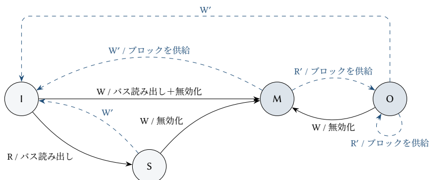
図 19.3: MOSI プロトコル。記法は図 19.2 と同じ。網掛けの状態は、主記憶より新しいブロックに責任を持つ。O での W' では、書き込んだコアがミスした場合にのみブロックが供給される。
