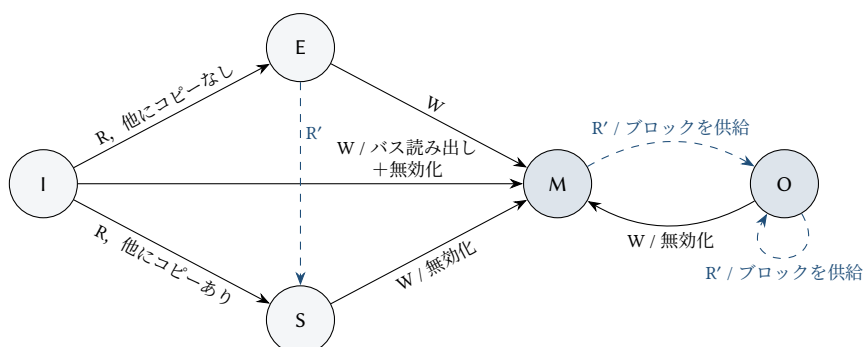
図 19.4: MOESI プロトコル. 記法は図 19.2 と同じ. I から出るすべての遷移はバス読み出しを行う. 他のコアによる書き込みは, すべての有効な状態を I へ移す. 書き込んだコアがミスした場合は, M または O のキャッシュがブロックを供給する (これらの辺は描いていない).
