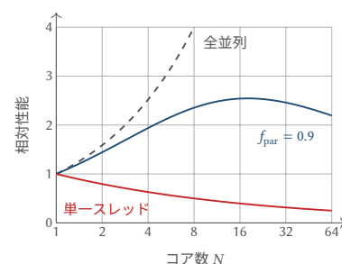
図 22.3: 1 コア分の電力バジェットを N 個のコアが分け合うときの性能。式 (22.3) による。
