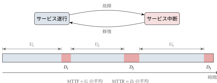
図 17.2: 2つのサービス状態と、それらを交互に繰り返す履歴。 U_i がサービス遂行の期間、 D_i がサービス中断の期間である。
