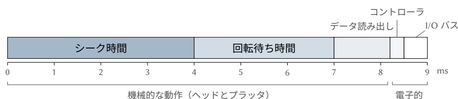
図 16.2: 例 16.2 のアクセスを実寸で描いたもの。9 ms のうち 8.2 ms を機械的な動作が占める。
