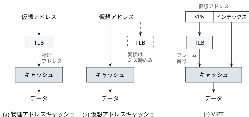
図 14.2: TLB とキャッシュ探索を組み合わせた 3 つの方法. (b) では変換はミス時にだけ必要なので, TLB はヒットの経路に入らない (権限の確認のためには依然として参照される). (c) では, インデックスがすでにセットを選んでいる間に TLB が仮想ページ番号を変換する.
