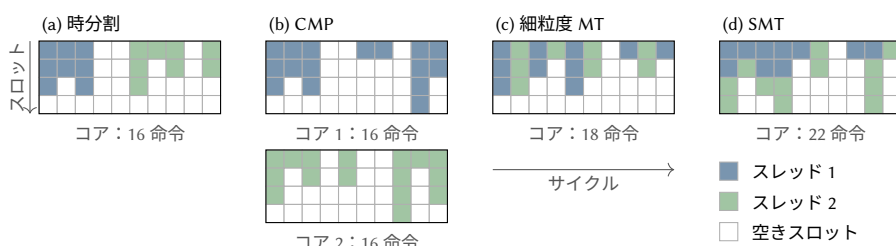
図 18.4: 2つのスレッドによる、コアのサイクル当たり 4 スロットの 10 サイクルにわたる使われ方の模式図。各列が 1 サイクル、各行が 1 スロットである。単独ではどちらのスレッドもこの 10 サイクルで 16 命令を実行する (b)。(a) は 5 サイクルごとにスレッドを切り替え、(c) は待っていないスレッドの間で交互に切り替える。
