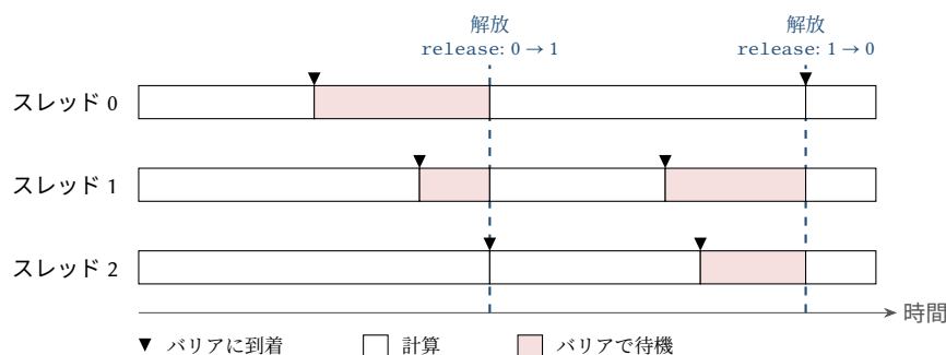
図 20.3: 3 つのスレッドが連続する 2 回のラウンドで使うバリア。各ラウンドは、そのラウンドの最後のスレッドが到着した時点で解放される。
