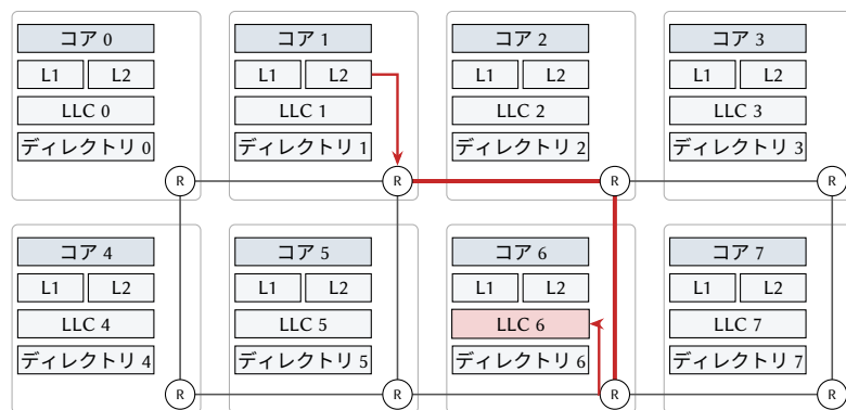
図 22.2: メッシュで接続された 8 つのタイル。各タイルはコア、その L1 と L2 キャッシュ、分散 LLC の 1 スライス、オンチップディレクトリの一部（22.4 節）、そしてルータ (R) を保持する。セット番号が 2 進で 110 で終わるブロックに対するコア 1 の L2 ミスは、LLC スライス 6 へ送られる。
