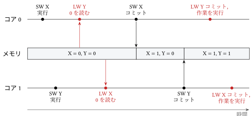
図 21.1: 2つのアウトオブオーダーコア上での例21.2。各コアのロードは自分のストアがコミットする前にメモリを読み、両方のロードが0を読んで、両方のコアが作業を行う。
