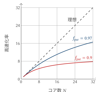
図 18.1: N コアでの高速化率: 理想的なスケールと式 (18.1).
