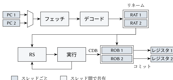
図 18.5: 2 つのスレッドのための SMT を備え、ROB を分離したアウトオブオーダーコア。ROB を共有する場合、スレッドごとに保持されるのはプログラムカウンタ、RAT、アーキテクチャレジスタだけである。
