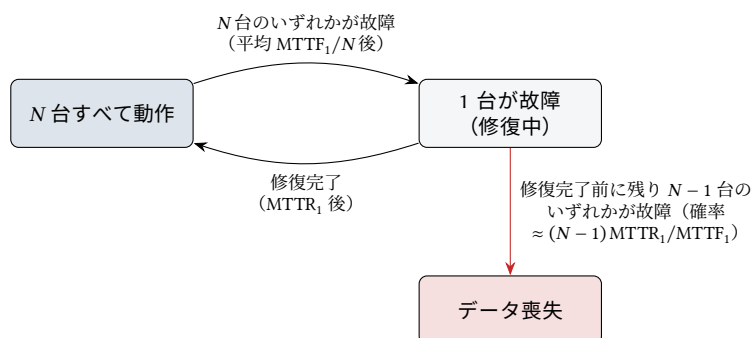
図 17.5: 1 台のディスク故障を許容するアレイと、その修復。データが失われるのは、1 台目を修復している間に 2 台目が故障した場合だけである。RAID 1 では N = 2 である。
