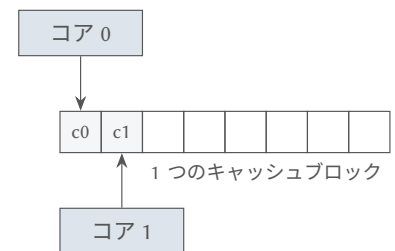
図 19.6: 偽共有: 異なるコアが使うカウンタが同じキャッシュブロックにある。
