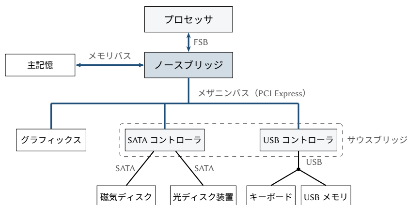
図 16.4: バスの階層。グラフィックスアダプタはメザニンバスに直接接続される。ディスクなどのより遅いデバイスには、メザニンバス上の SATA コントローラと USB コントローラを介して到達する。これらのコントローラはより遅い標準 I/O バスを提供する。PC のチップセットでは、これらのコントローラがサウスブリッジ（破線）をなす。
