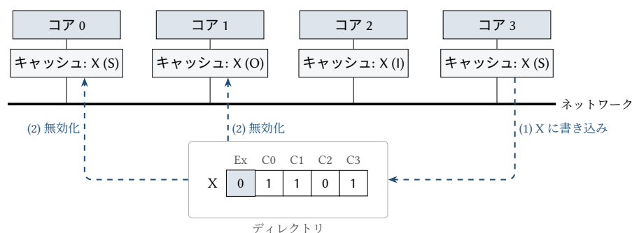
図 19.5: 例 19.10 の手順 5 におけるディレクトリ方式. X のエントリは, コア 0, 1, 3 がコピーを保持しており, どのコアも X を排他的には保持していないことを示す. コア 3 の書き込み (1) は, コア 0 と 1 だけへ無効化として転送される (2).
