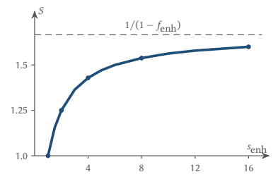
図 2.1: f_{\text{enh}} = 0.4 のときの全体の高速化率 S . 改善部分が速くなるほど, 同じ部分をさらに改善して得られる効果は小さくなる.
