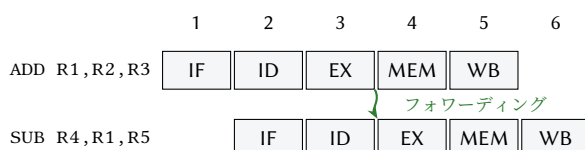
図 3.4: フォワーディング: ADD の ALU 結果を SUB の EX ステージへ直接送り、ストールを回避する。
