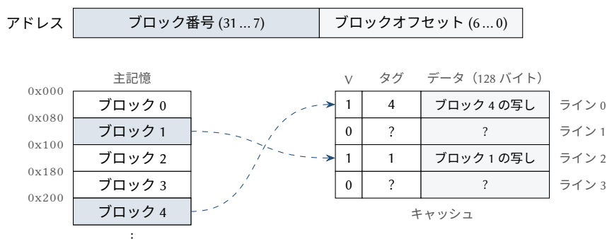
図 12.2: 128 バイトのブロックに分割された主記憶と, 4 ラインのキャッシュ. ライン 0 と 2 はブロック 4 と 1 の写しを保持し, ライン 1 と 3 は有効なものを何も保持していない.
