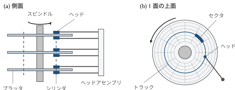
図 16.1: 磁気ディスクの構造。 (a) スピンドル上のプラッタと、1 面につき 1 つのヘッド。すべてのヘッドのアームはヘッドアセンブリをなし、破線は 1 つのシリンダを示す。 (b) 1 つの面。同心円状のトラックに分けられ、各トラックはセクタに分けられる。1 つのトラックとそのセクタの 1 つを強調してある。
