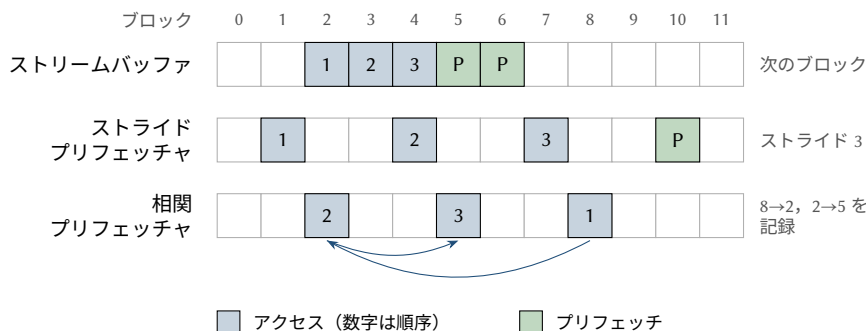
図 14.5: 3 つのハードウェアプリフェッチャが利用するアクセスパターン。図示した 3 回のアクセスの後、ストリームバッファは続くブロックを、ストライドプリフェッチャは 1 ストライド先のブロックを取得し、関連プリフェッチャは次にブロック 8 がアクセスされたときにブロック 2 を取得する。
