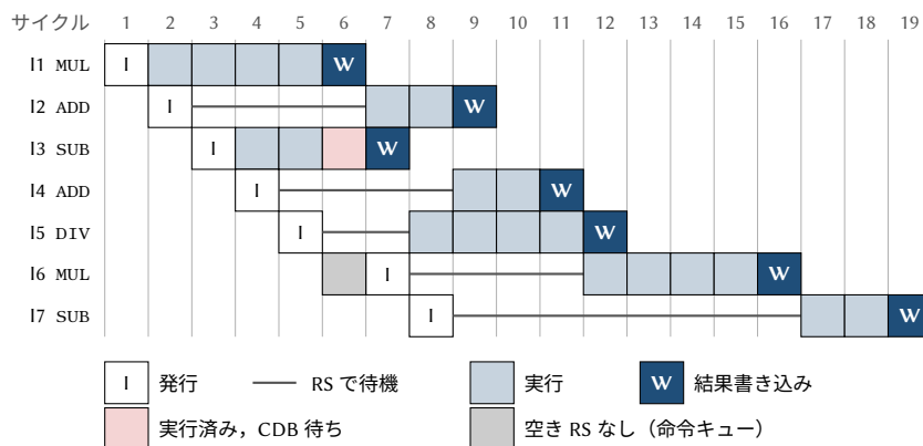
図 7.4: 実行例のタイミング. アウトオブオーダ実行により, I2 が待っている間に I3 が実行され, I4 が待っている間に I5 が実行を始める. I3 (バス), I4 (加減算器), I6 (リザベーションステーション) の遅延は, 例 7.7 で導いたものである.
