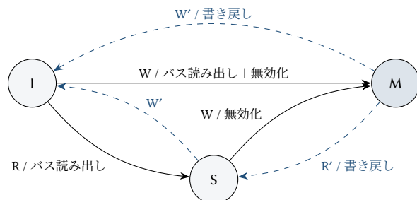
図 19.2: 1 つのキャッシュ内の 1 つのブロックに対する MSI プロトコル。R, W はこのコアによる読み出しと書き込み、R', W' (破線) はバス上で観測される他のコアによる読み出しと書き込みである。辺のないアクセスは状態を変えず、バス操作も必要としない。網掛けの状態は、主記憶より新しいブロックを保持している。
