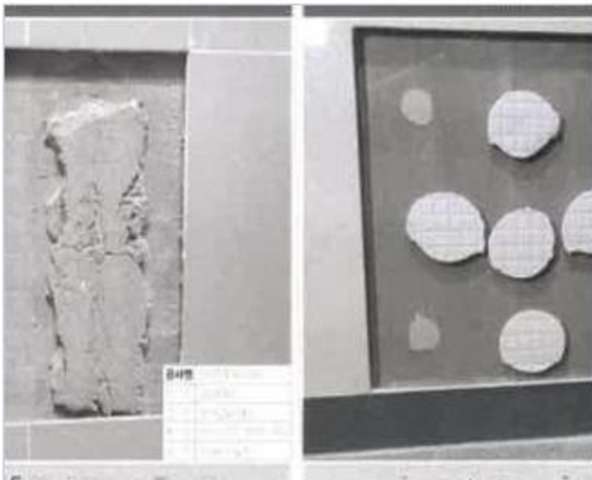
타일 탈락면 · 뒤풀음 부족 상태 (타 단지 조사 사진)
