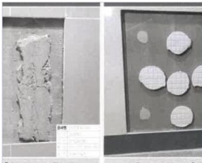
타일 탈락면 · 뒤편 부족 상태 (타 단지 조사 사진)
