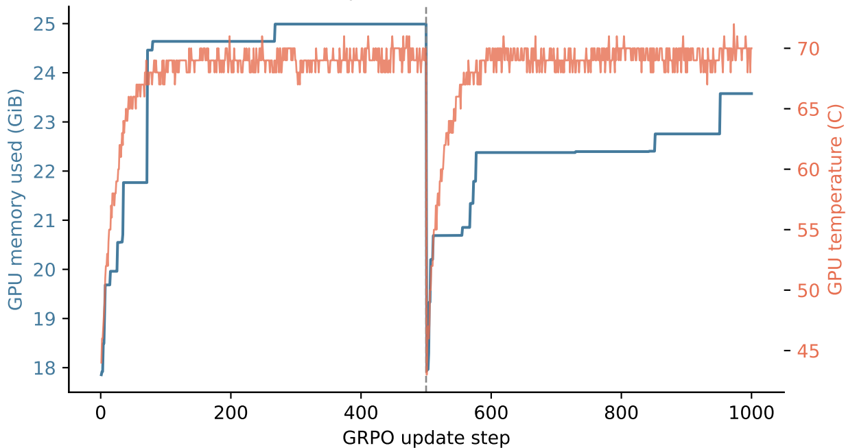
Resource profile on RTX 6000 Ada
