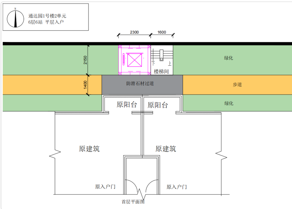
【图1】电梯改造一层平面方案图
