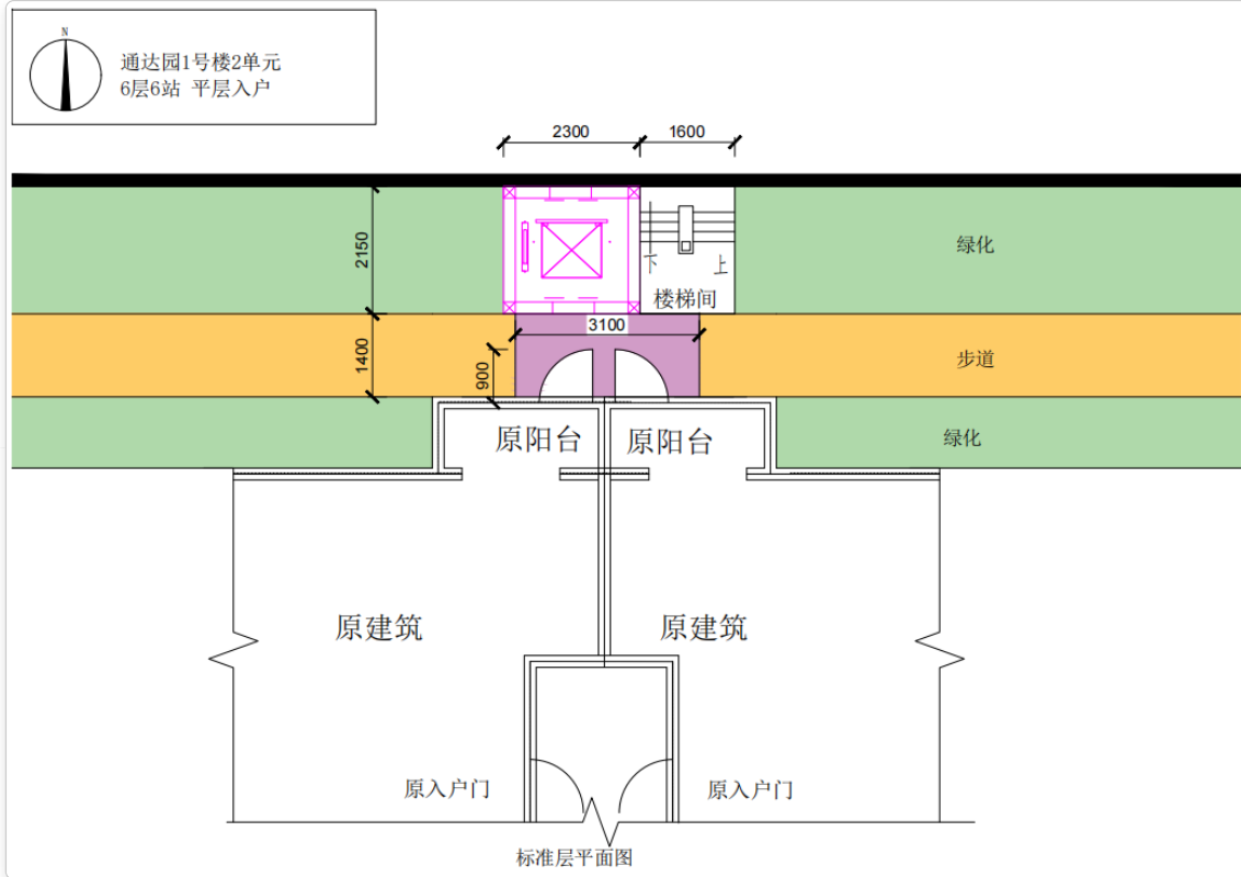
【图2】电梯改造二层以上方案图
