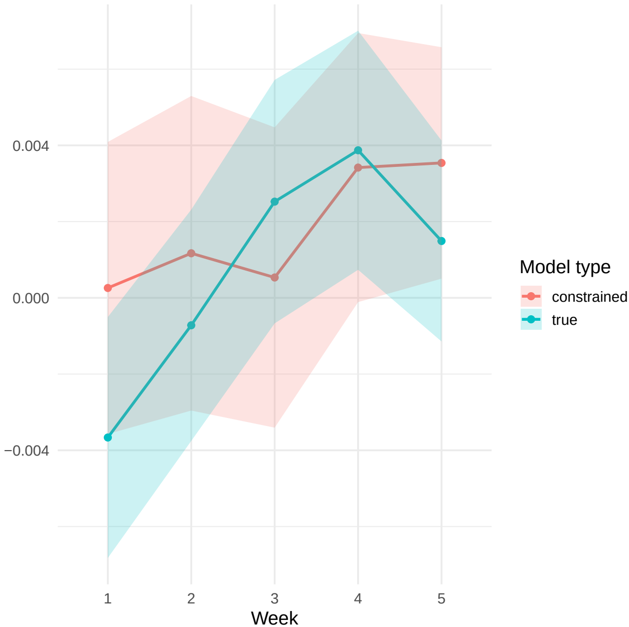
Parameter estimates over time: nonconformity
