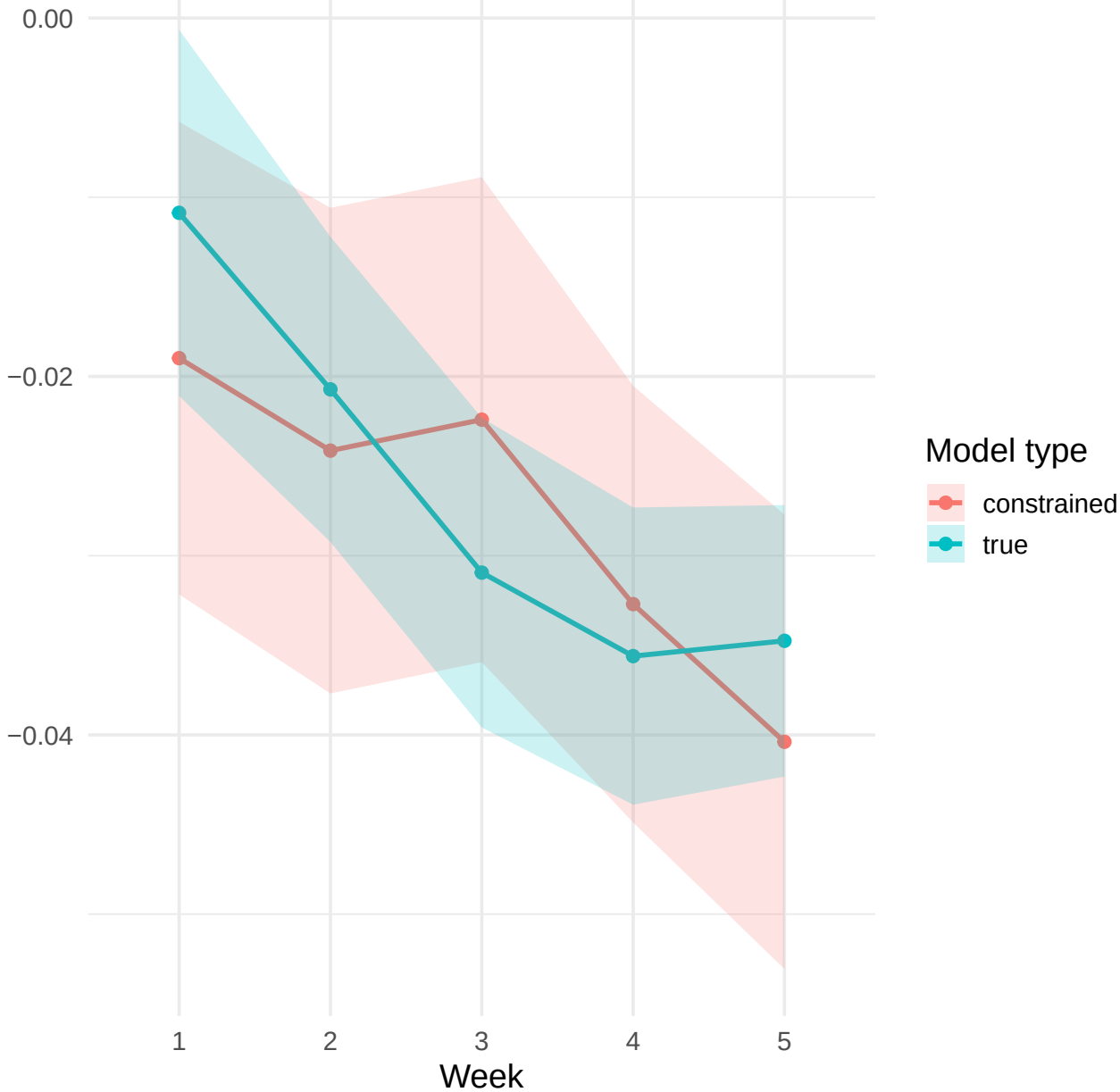
Parameter estimates over time: nonconformity.localAND
