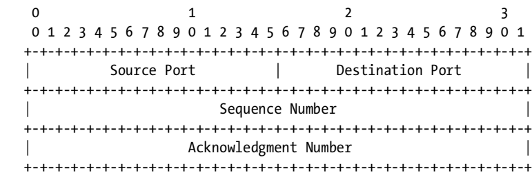
TCP Header Format
