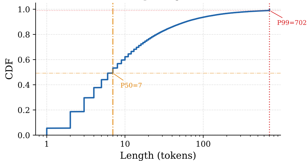
(d) Output Length CDF
