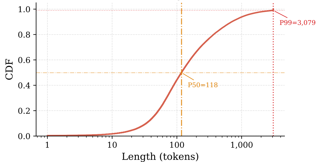
(d) Output Length CDF
