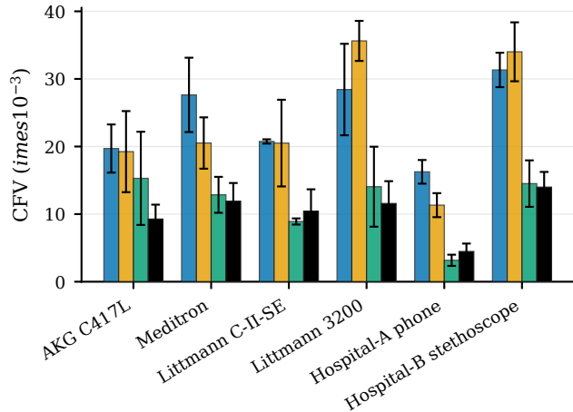
(b) CFV
