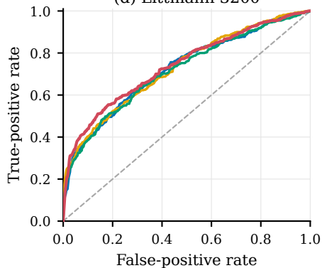
(d) Littmann 3200
