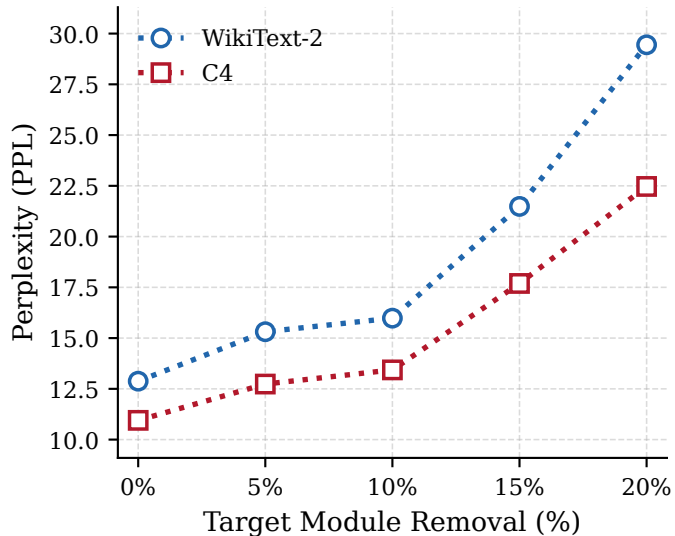
(b) Llama-3.1-8B-Instruct
