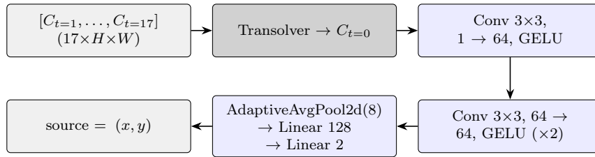
Рис. 7: Архитектура Transolver + регрессия координат
