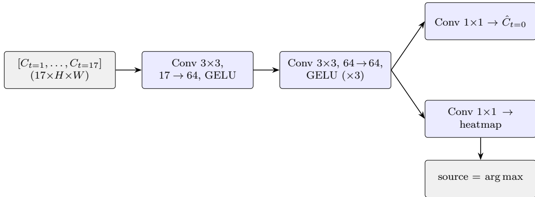
Рис. 15: Архитектура PINN: свёрточная сеть с двумя головами (поле и heatmap)
