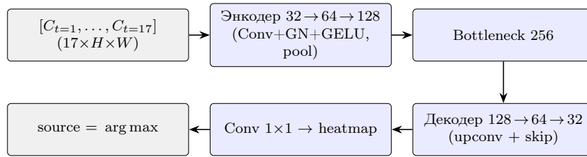
Рис. 11: Архитектура UNet + heatmap
