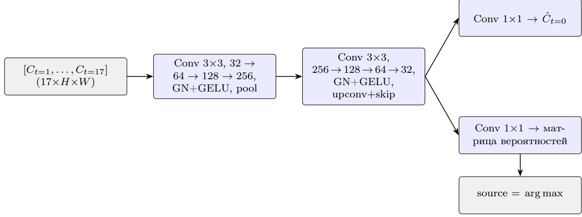
Рис. 11: Архитектура UNet с двумя головами
