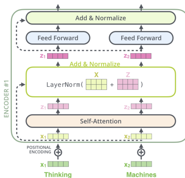
Рис.2.7. Слои Add & Norm подробно [3]
