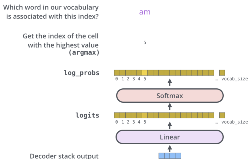
Рис.2.10. Слои Linear и Softmax [3]
