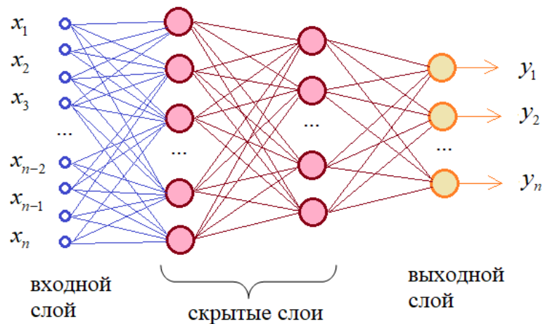
Рис.2.9. Полносвязная нейронная сеть (Feed-Forward Neural Network) [3]
