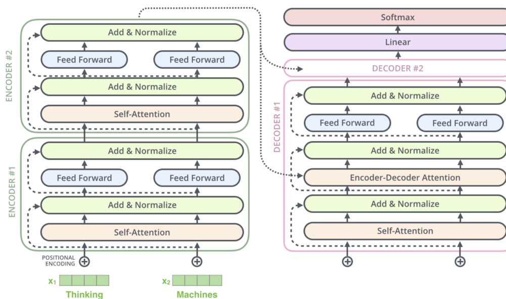
Рис.2.8. Подробная архитектура Transformer [3]
