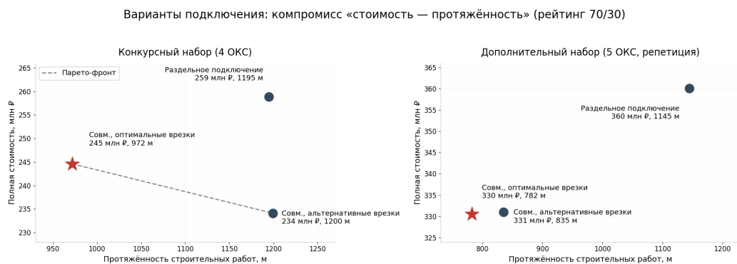
Рис. 1 — Варианты на плоскости «стоимость — протяжённость»; звёздочкой отмечен рекомендуемый (рейтинг 70/30)
